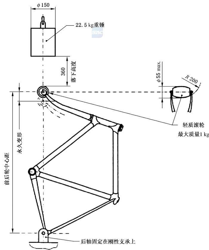
图 A.1 冲击试验(重物落下)
