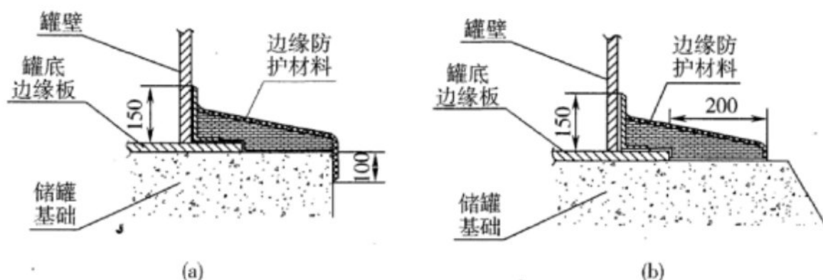
图 4.4.1 储罐罐底板边缘防护区域示意图
