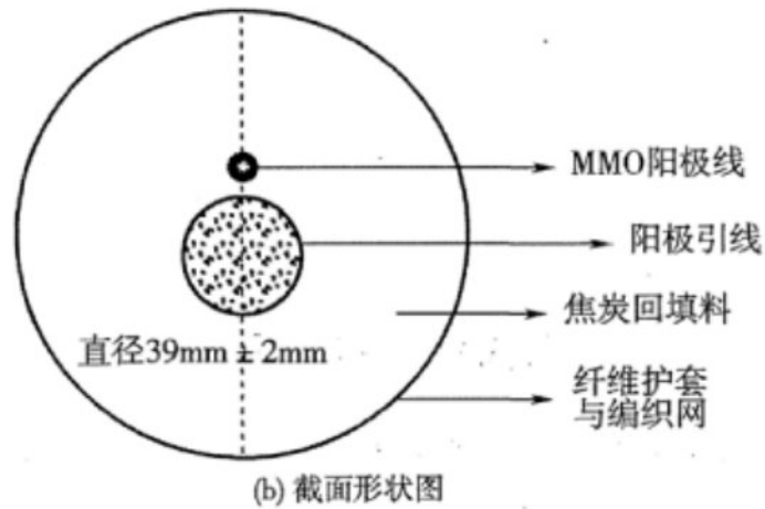
图 1 MMO/Ti 线性阳极示意图
