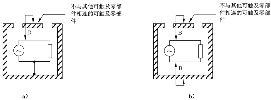
图 D.2a)和 b) 不与其它可触及零部件相连的可触及件对内部危险带电电路的防护
