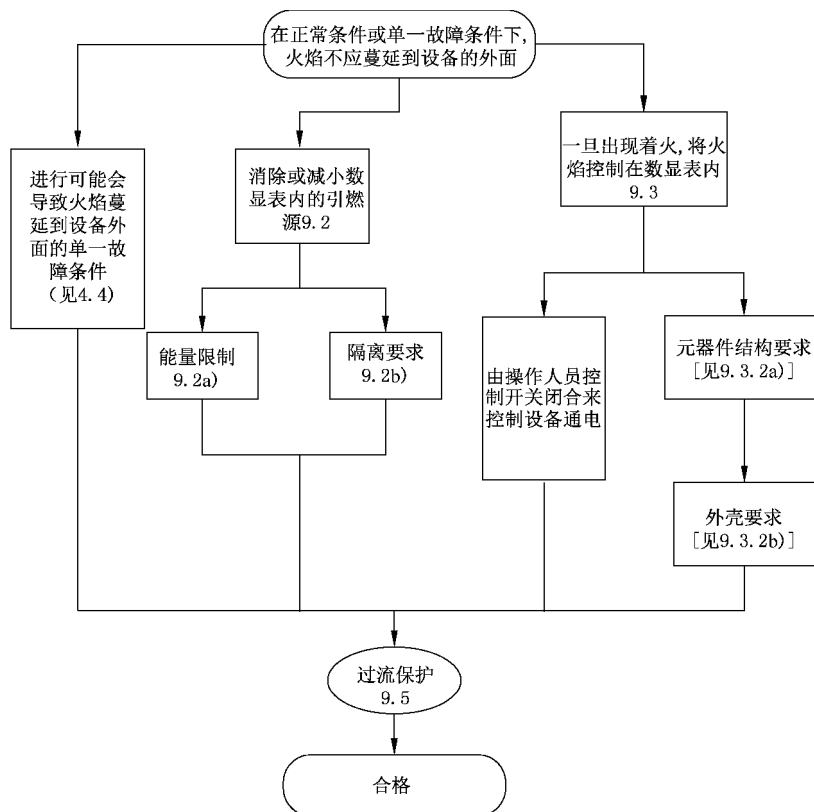
图 3 说明防止火焰蔓延要求的流程图
