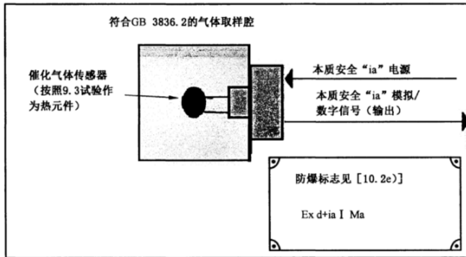
图7 Ma级“ia d”固定式监控传感器
