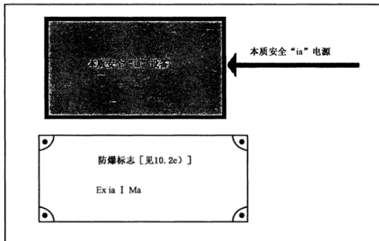
图 1 “Ma”级本质安全“ia”设备
