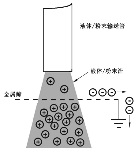
图 5 与流动绝缘物接触的危险接地导体
