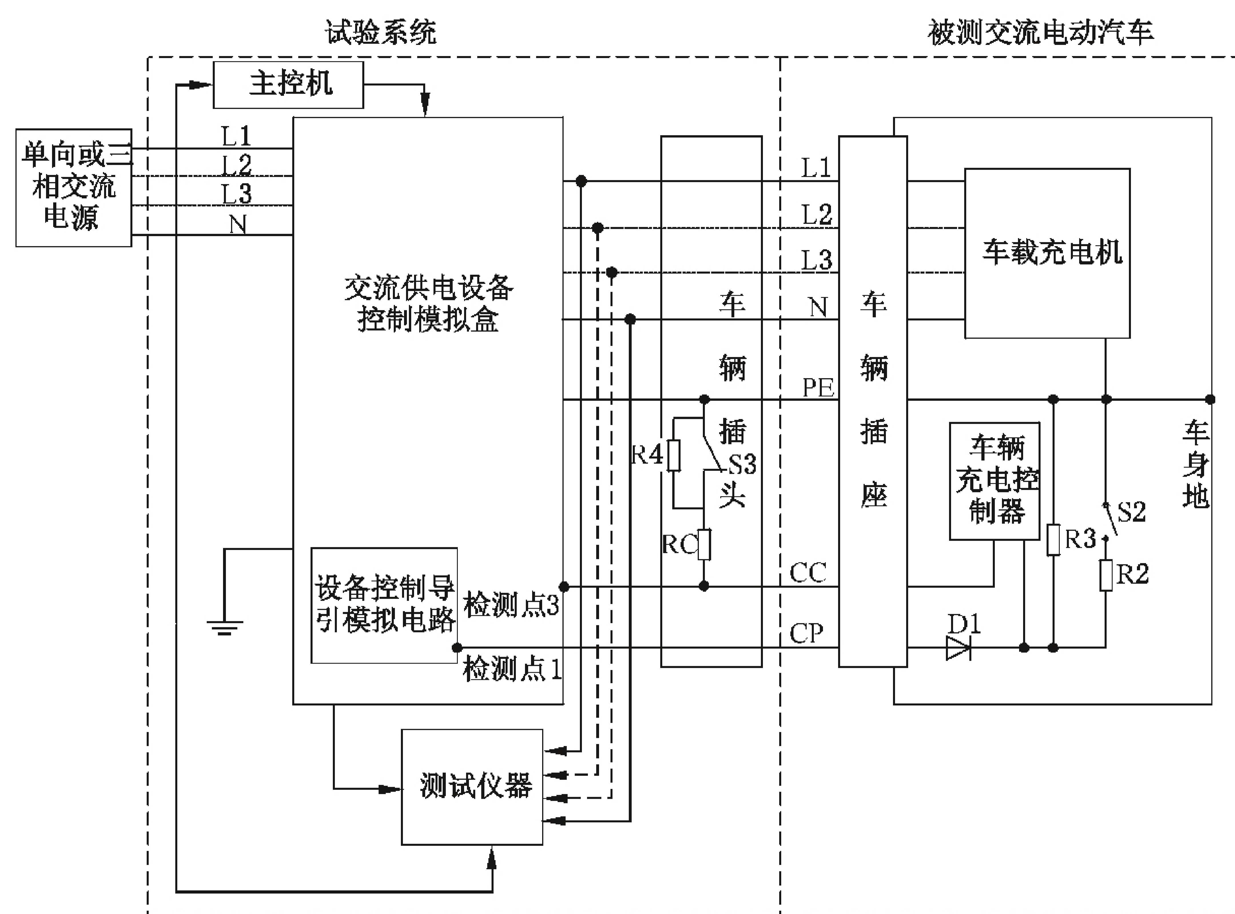
图4 电动汽车交流充电试验系统结构
