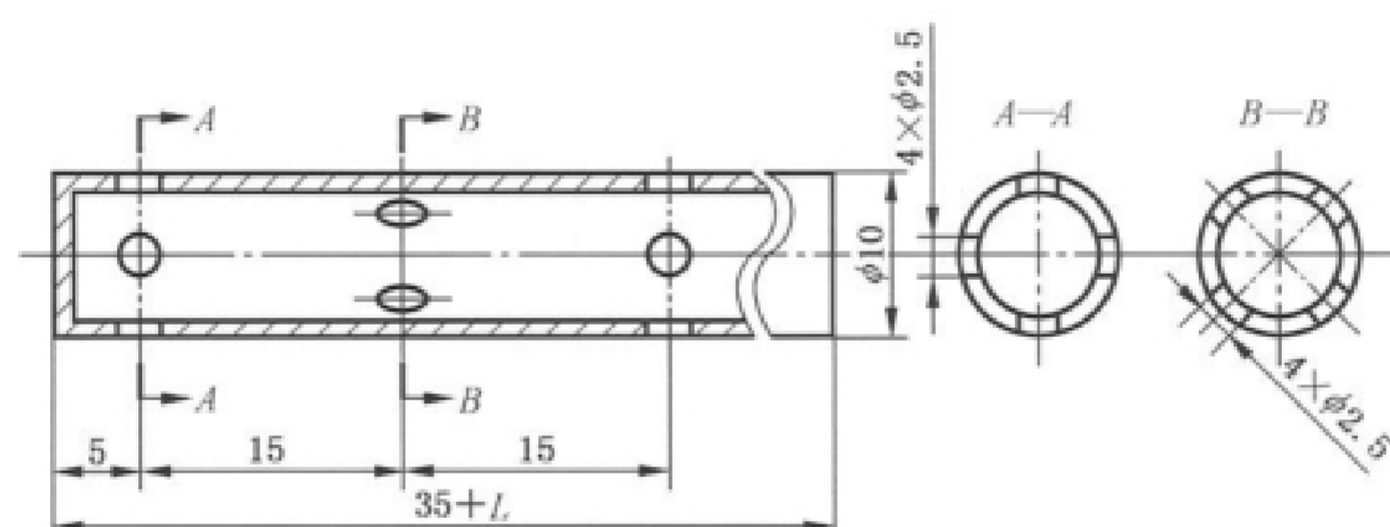
图5 烟管用取样器
