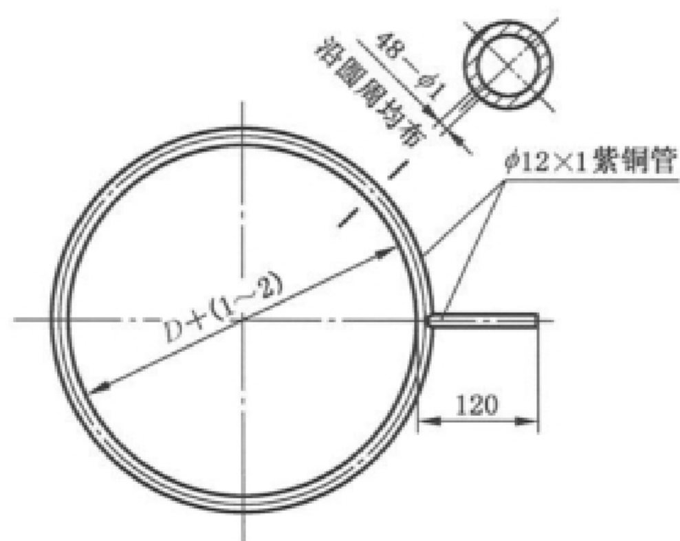
图 2 平底锅用取样器
