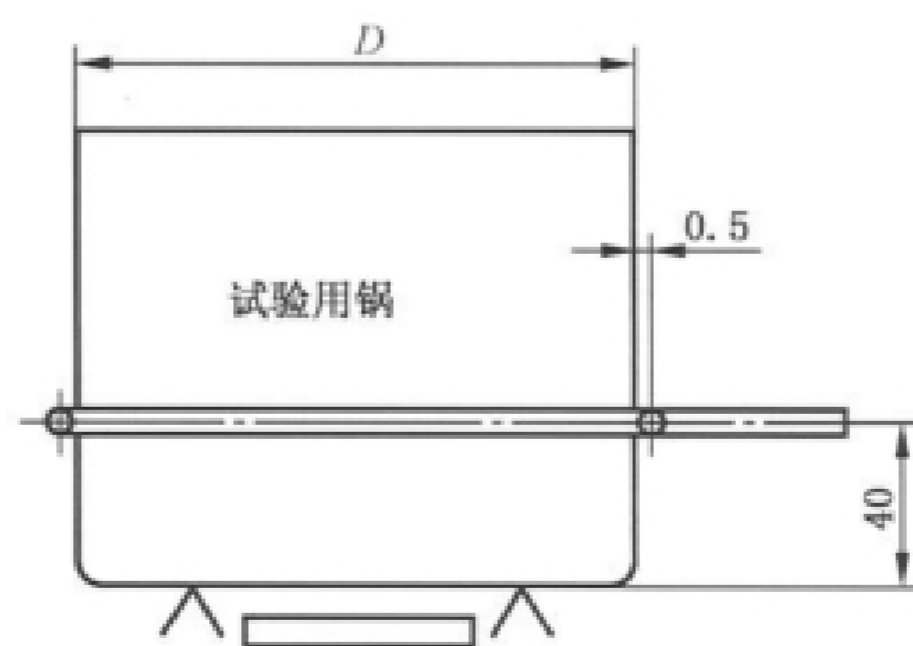
图 3 平底锅用取样器的安装位置
