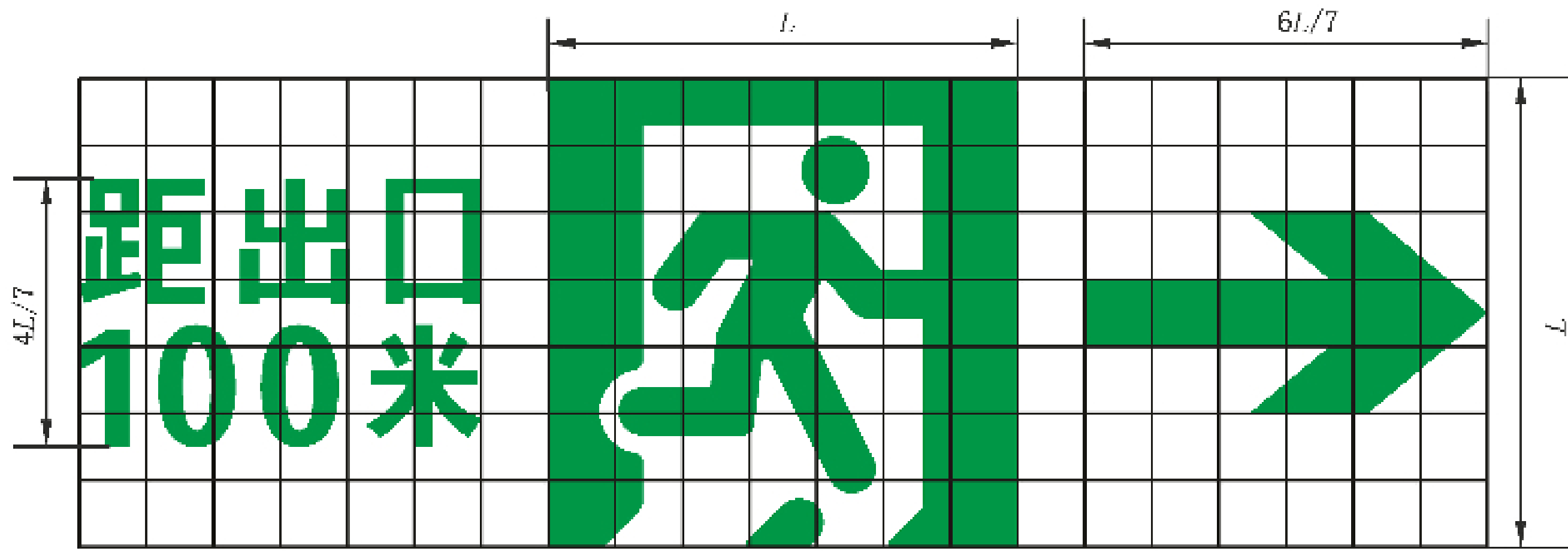
图 D.19 指示疏散出口距离标志图形
