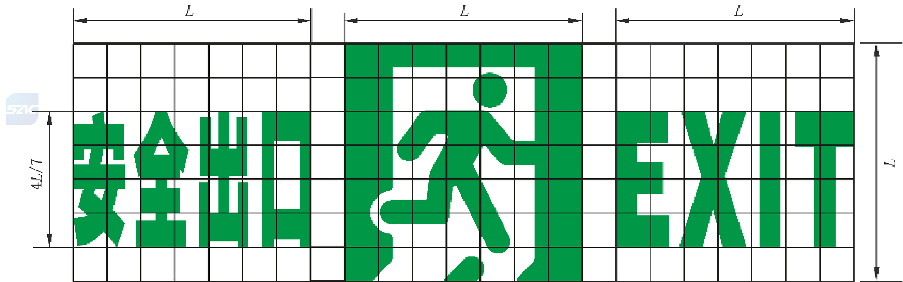
图 D.14 安全出口标志图形
