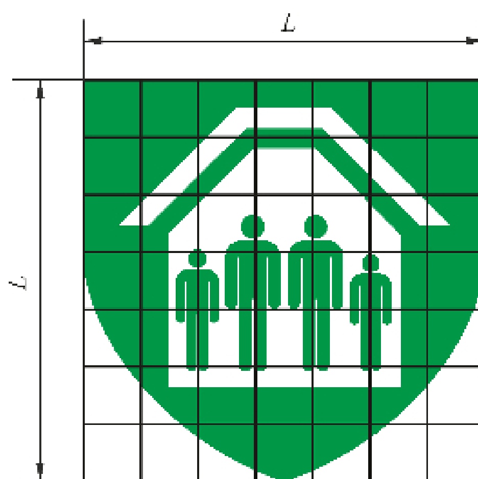
图 D.6 避难层标志图形
