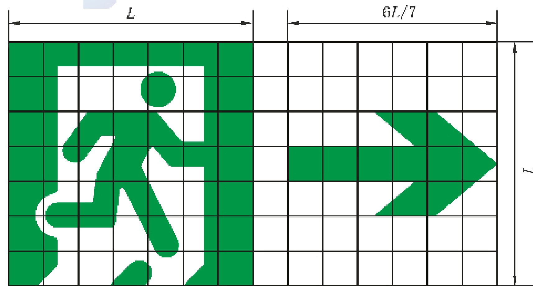
图 D.9 指示右向疏散标志图形
