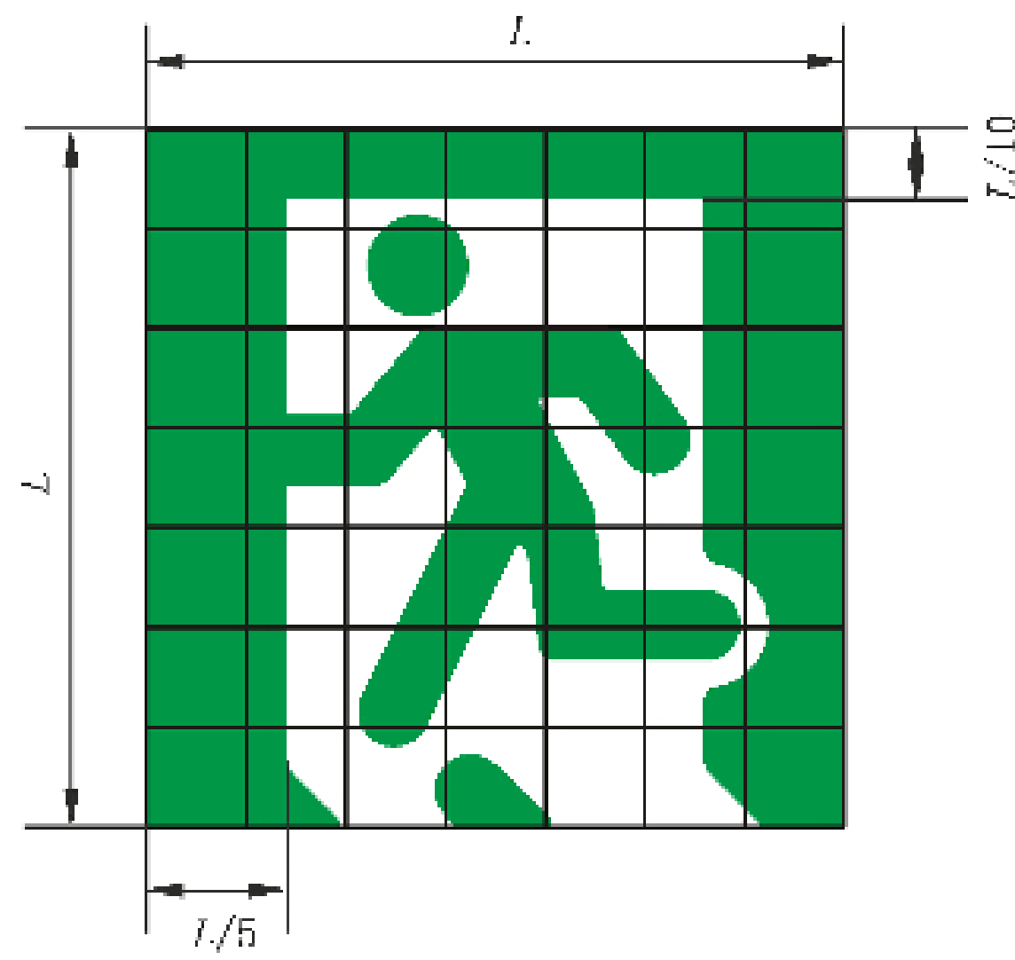
图 D.1 左向出口指示标志图形
