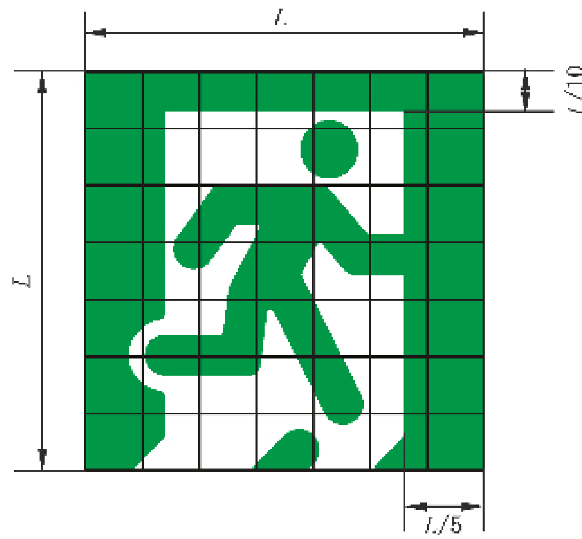
图 D.2 右向出口指示标志图形
