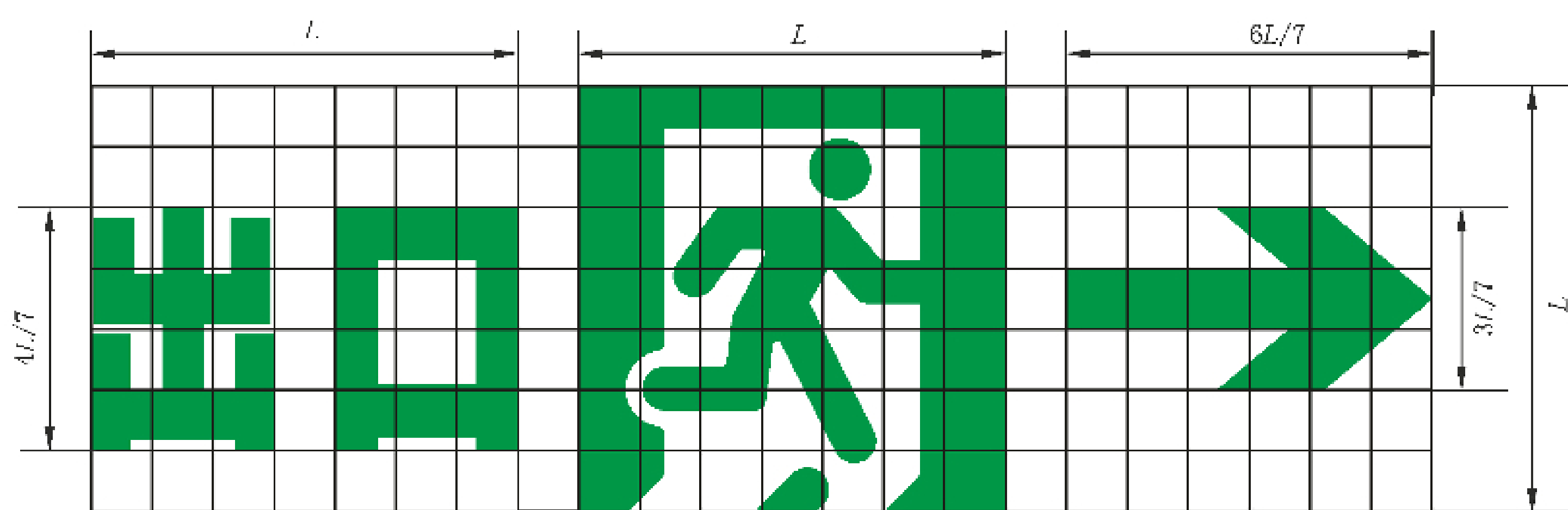
图 D.16 指示疏散出口方向标志图形
