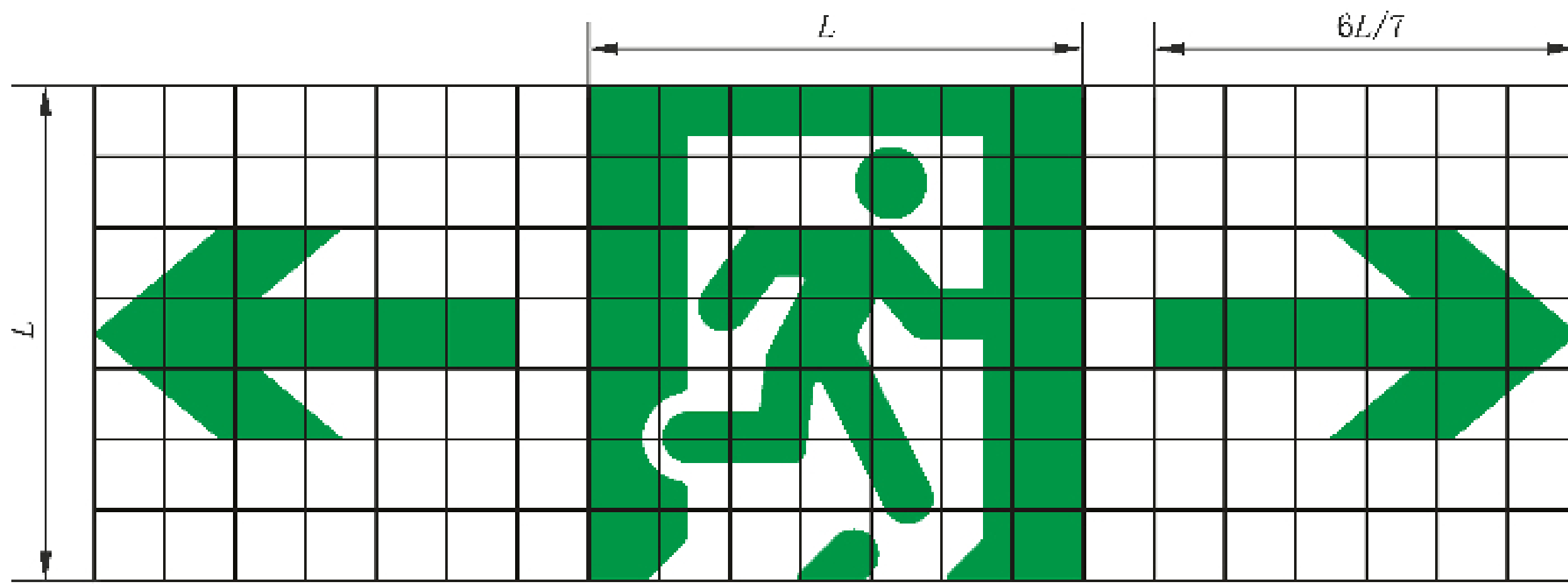
图 D.7 指示状态可变方向标志图形
