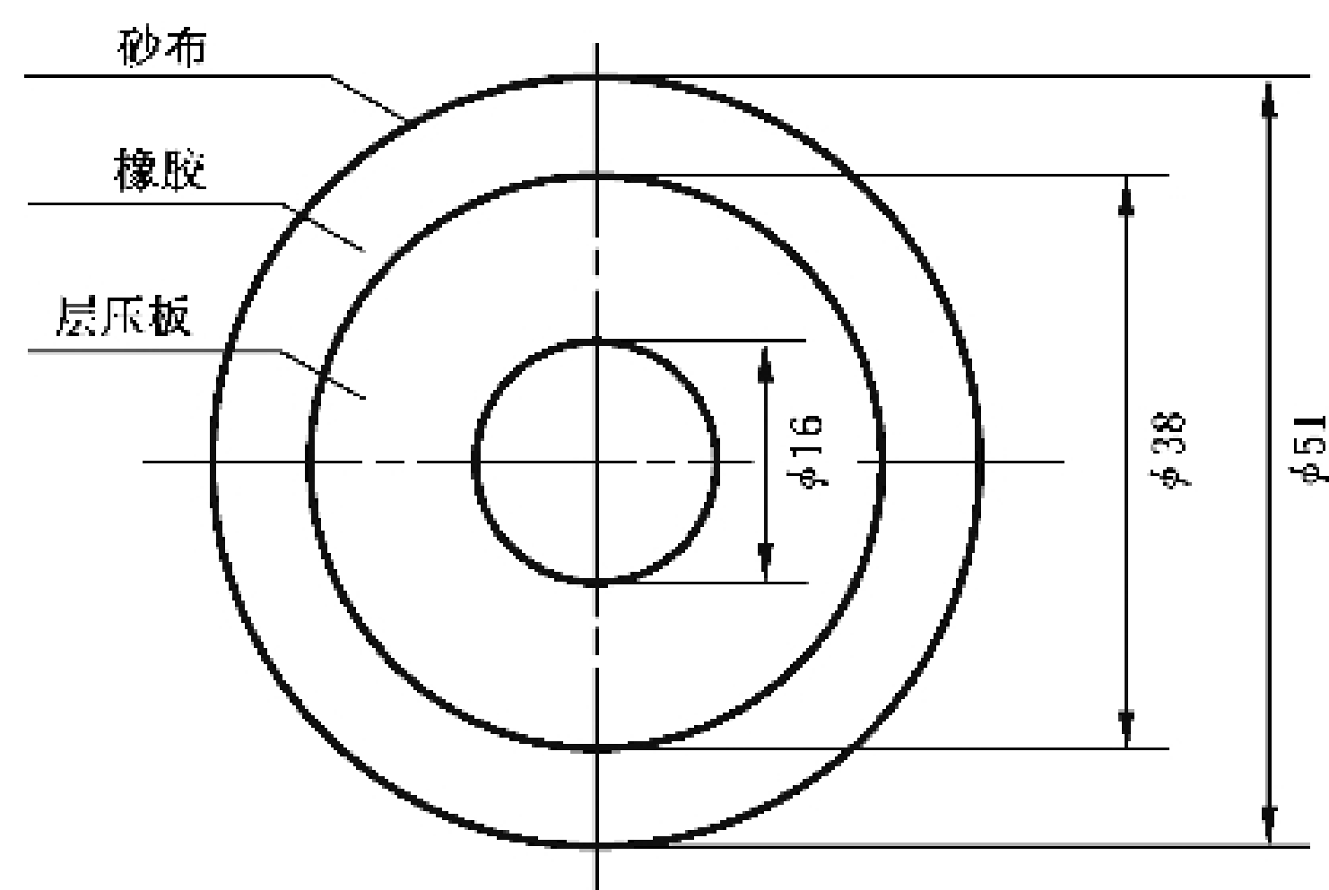
图 F.1 研磨轮
