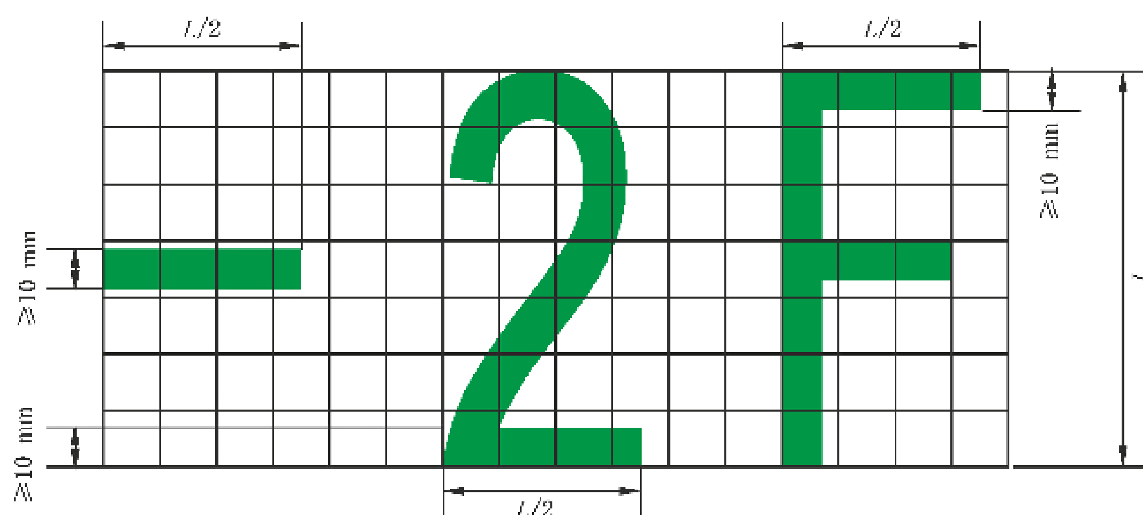
图 D.10 指示楼层指示标志图形
