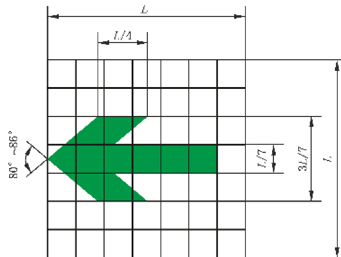
图 D.3 疏散方向指示标志图形
