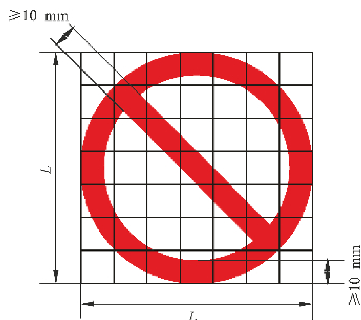
图 D.5 禁止入内标志图形
