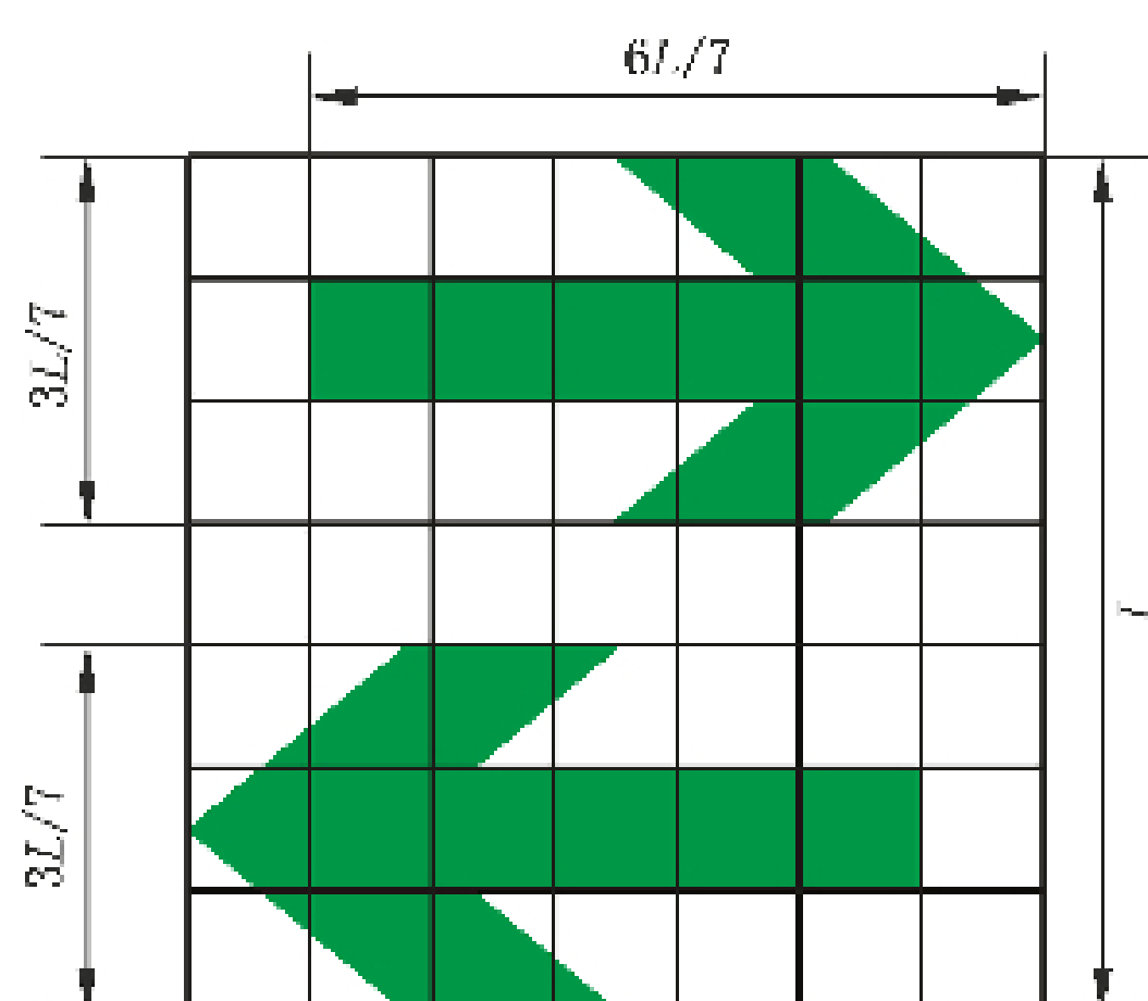
图 D.12 指示双向疏散标志图形
