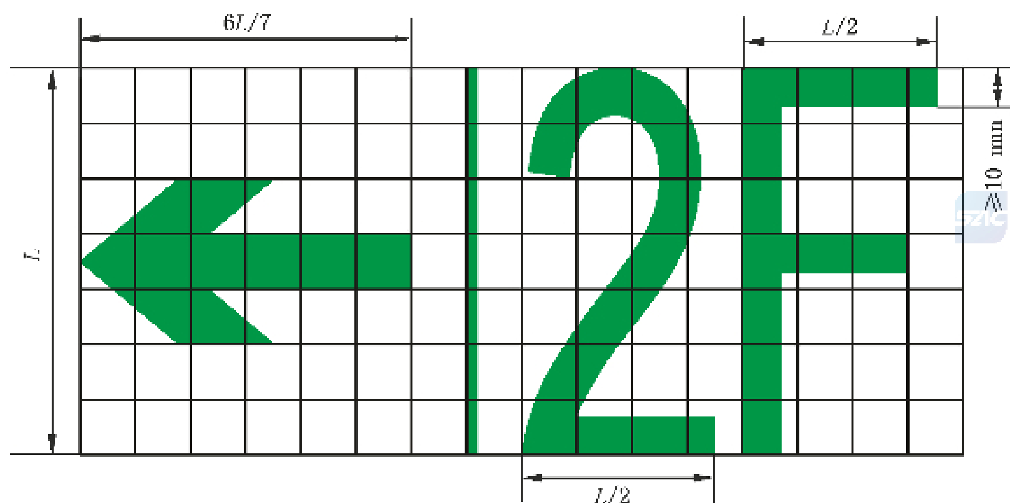
图 D.11 多信息复合标志图形
