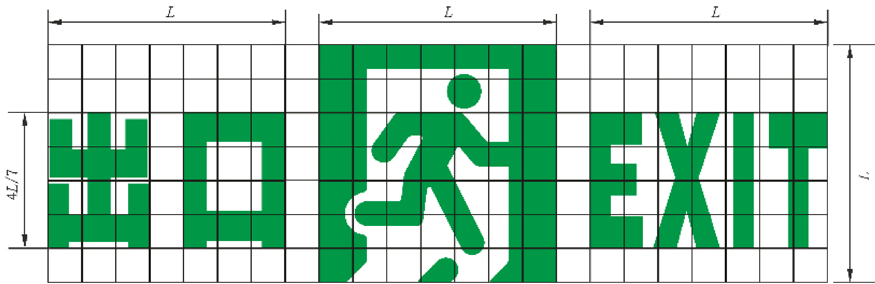
图 D.13 疏散出口标志图形
