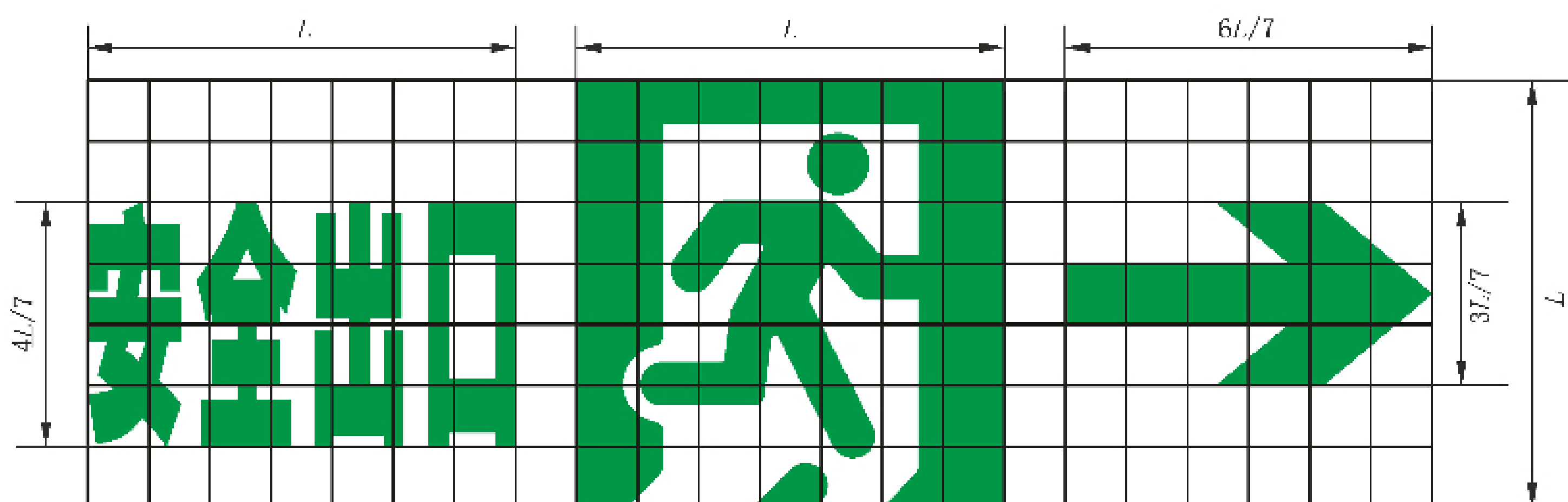
图 D.17 指示安全出口方向标志图形
