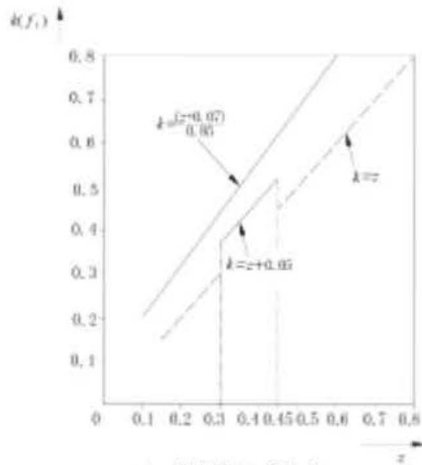
a) 特定的 N_1 类车辆
