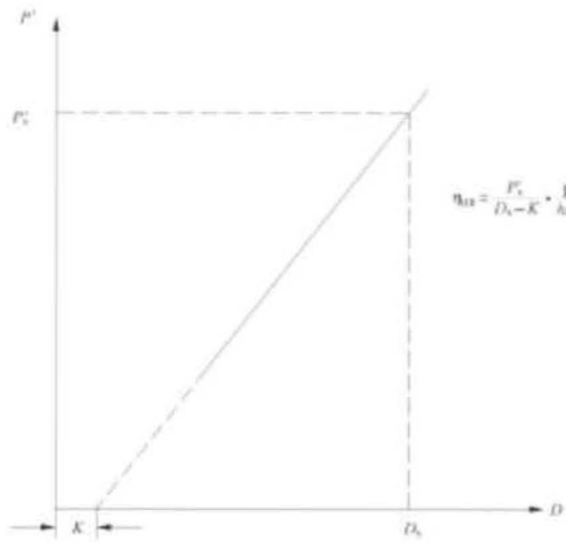
图 L.2 机械传输装置的 P'-D 关系曲线
