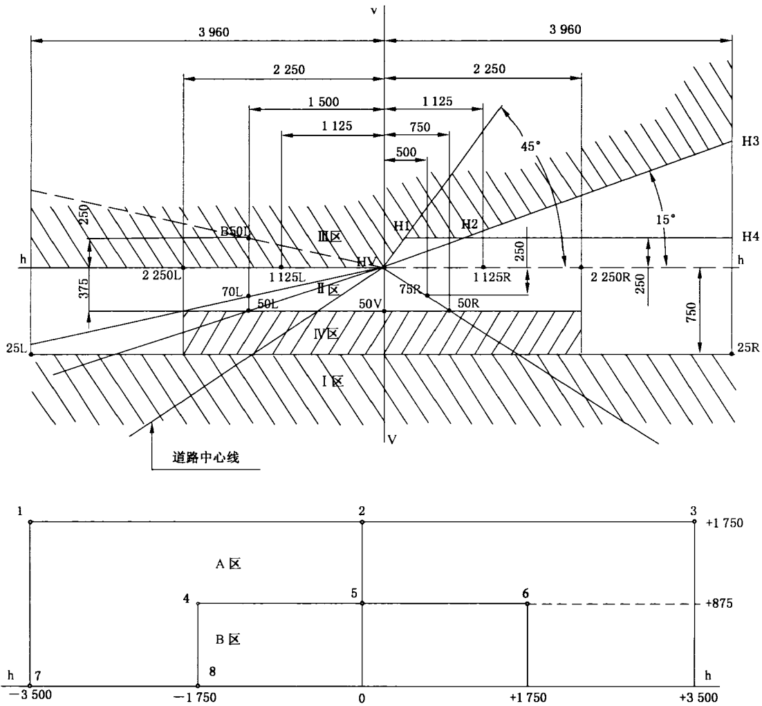
图 1 配光屏幕
