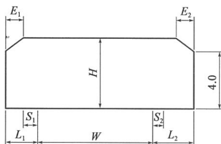
a) 高速公路、一级公路(整体式)
