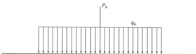
图 7.0.3 车道荷载
