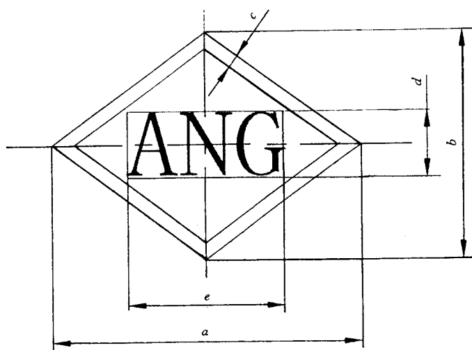
图 3 吸附天然气汽车标志图形
