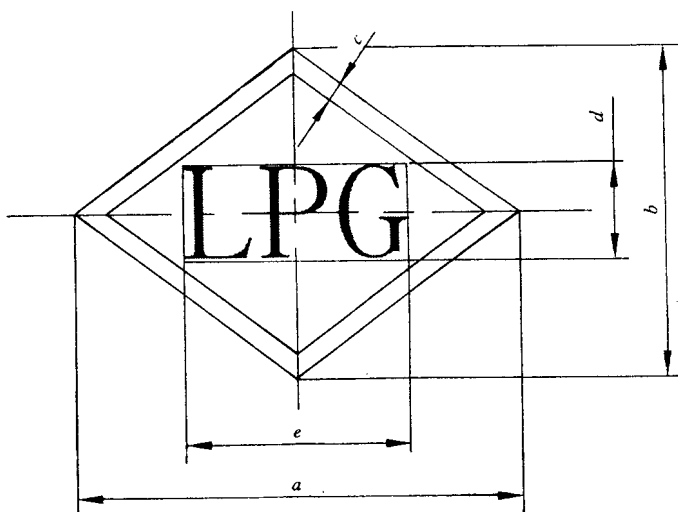
图 4 液化石油气汽车标志图形
