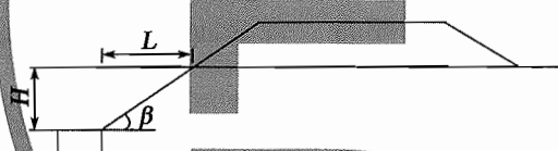
图7.6.3 溶洞安全距离(L)计算示意图
