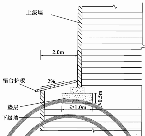
图 5.4.10 平台与垫层横断面图
