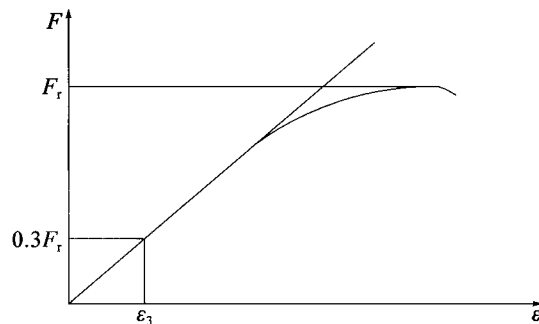
图 E. 4.4 荷载—应变曲线
