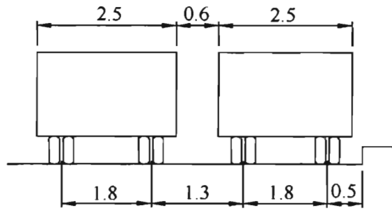
(6) 汽车荷载的横向布置
