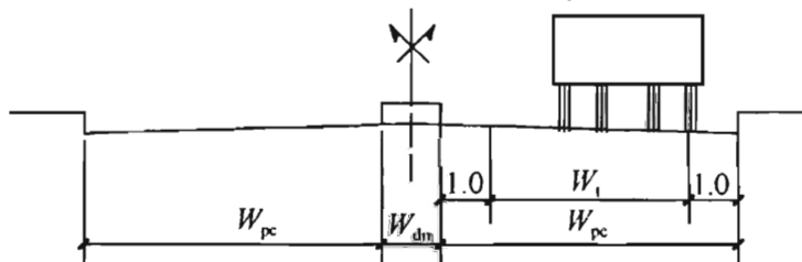
图 A.0.2-3 ( W_{pc} = 2 车道路面宽)
