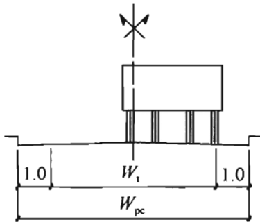
图 A.0.2-1 ( W_{pc} \leq 2 车道路面宽)
