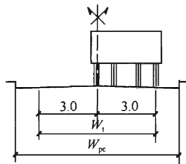
图 A.0.2-2 ( W_{pc} > 2 车道路面宽)
