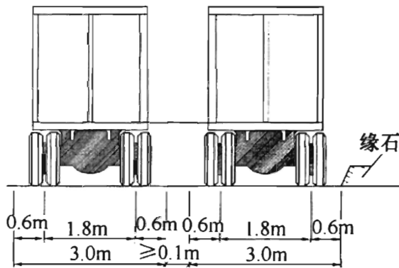
(6) 汽车荷载的横向布置
