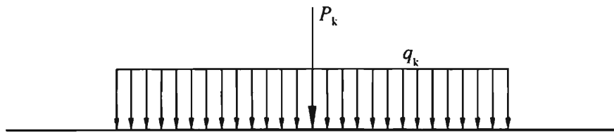
图 10.0.2-1 车道荷载
