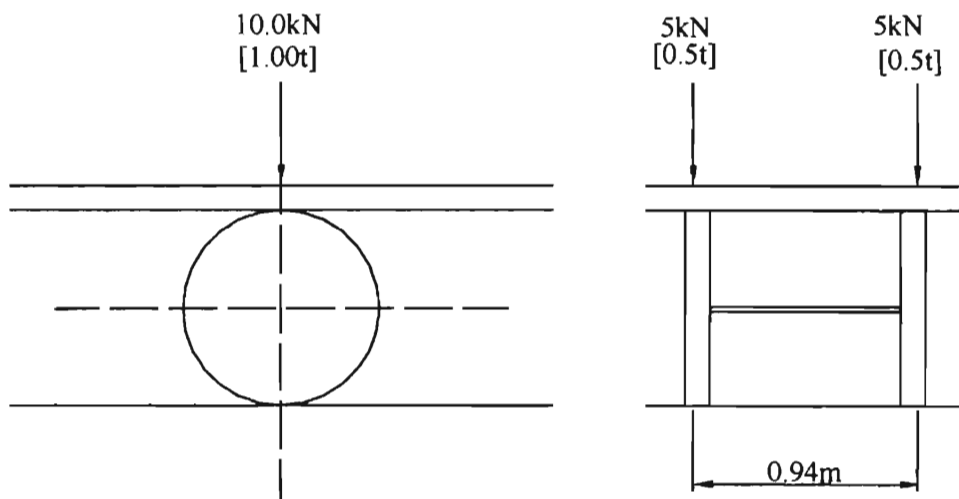
图 10.0.6 一辆人力劳动车荷载图
