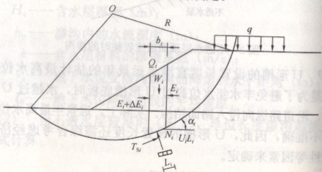
图 4 简化毕肖普法计算图示
