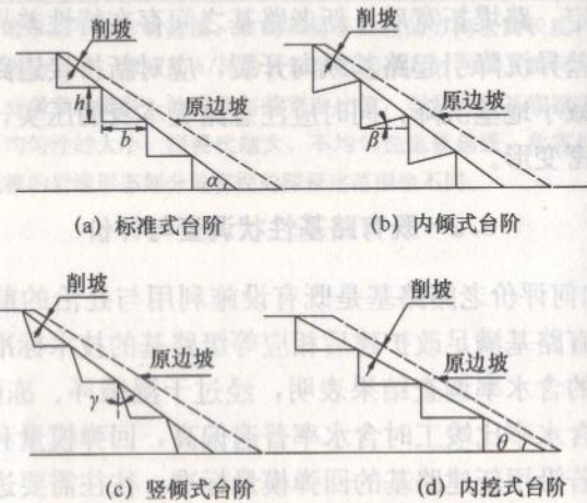
图6 台阶的基本形式
