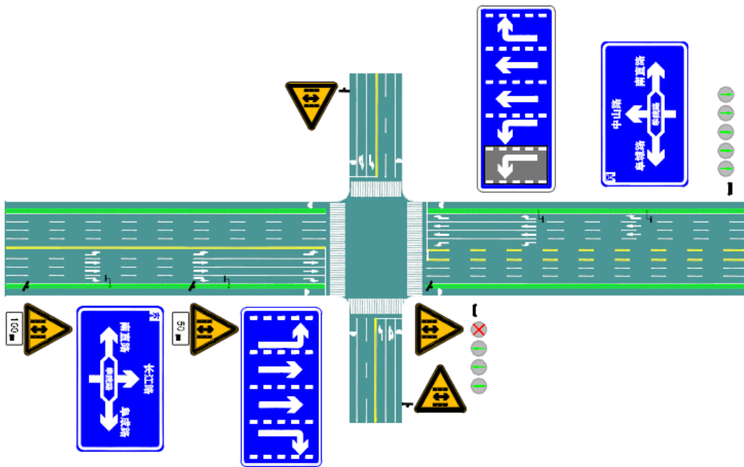
图 132 潮汐车道标志标线协调设置示例
