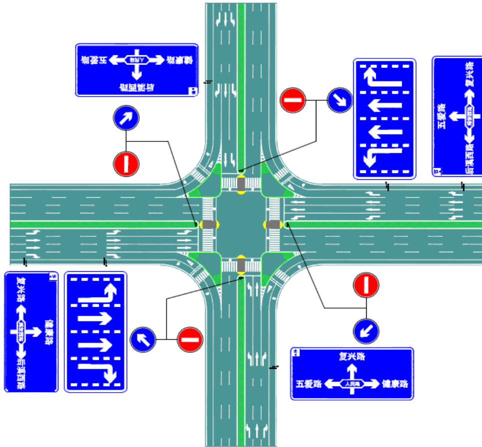
图 107 设置渠化岛的交叉口示例
