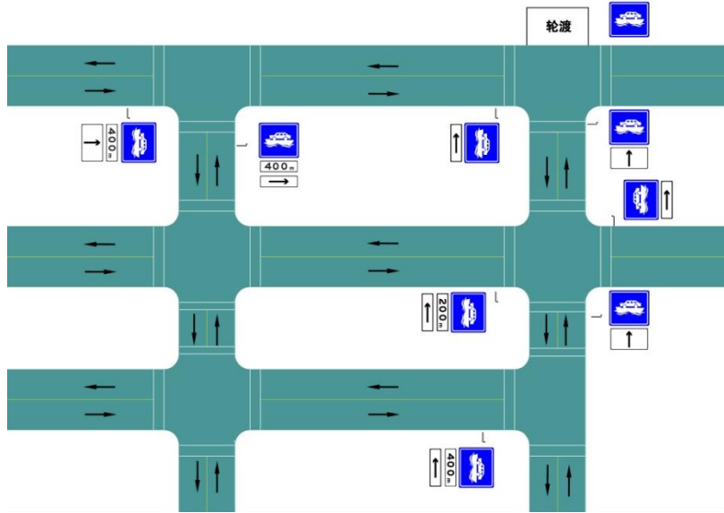
图 63 地点识别标志的设置
