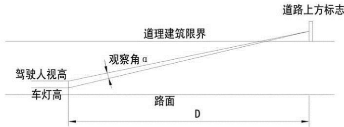
图 15 观测角
