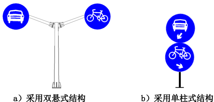
图 25 机非分隔带处专用道路和车道标志同杆设置
