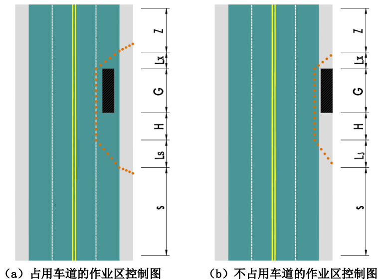
图 103 作业路段控制图
