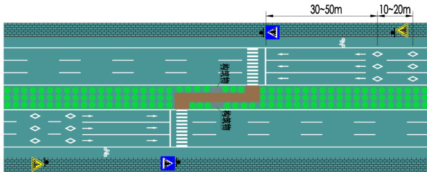
图 87 路段中人行横道线错位设置示例
