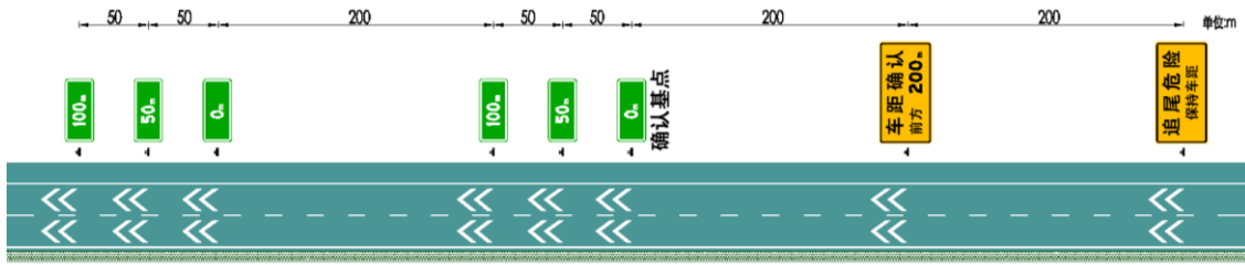
图 9.16.2 车距确认标志的设置
