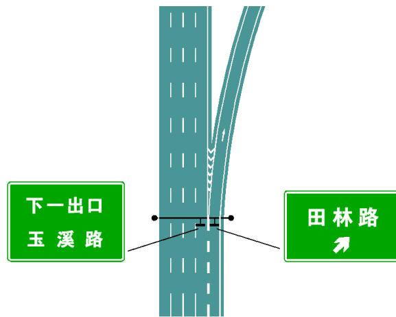
图 72 出口标志采用门架形式的设置
