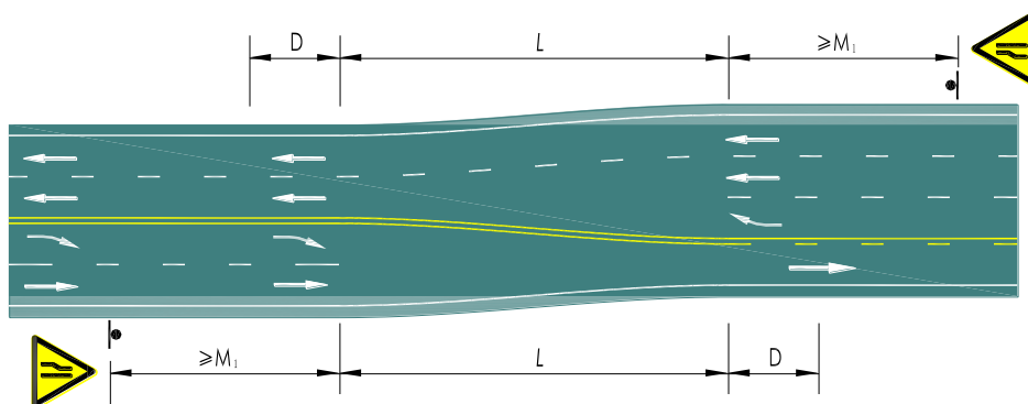
图 14.2.3 路面（车行道）宽度渐变段标线示例
