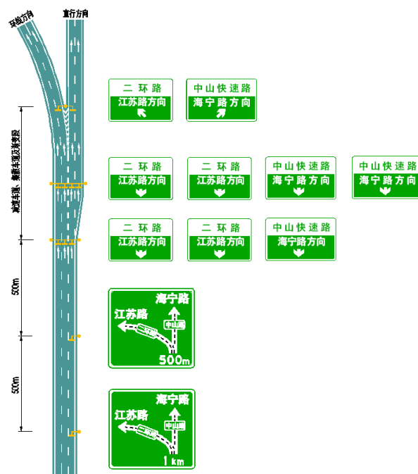
图 75 快速环线转向交通及直行交通均作主线指引的设置
