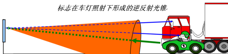
图 16 不同车辆驾驶人眼高区别
