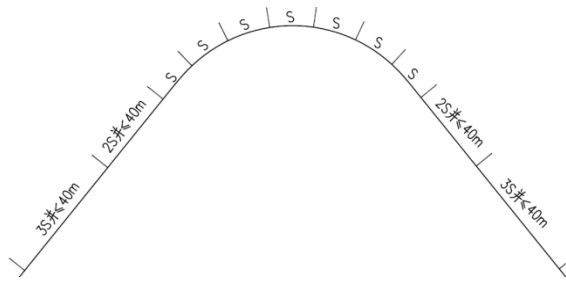
图 102 曲线段轮廓标设置间隔示例
