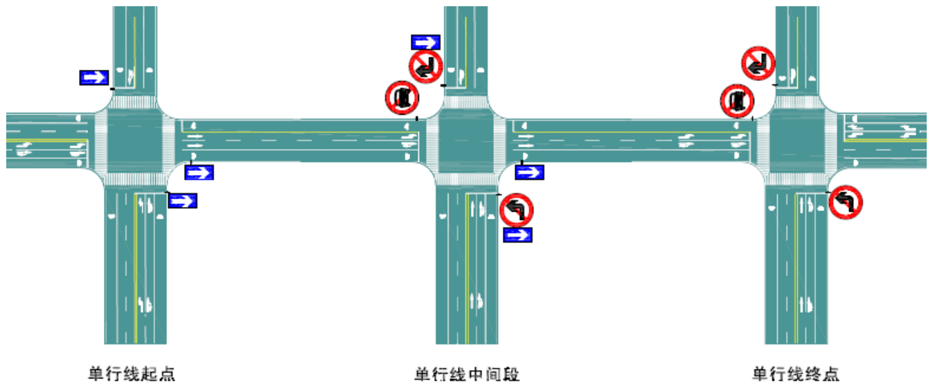
图 115 单行道起点、终点及中间段交叉路口示例
