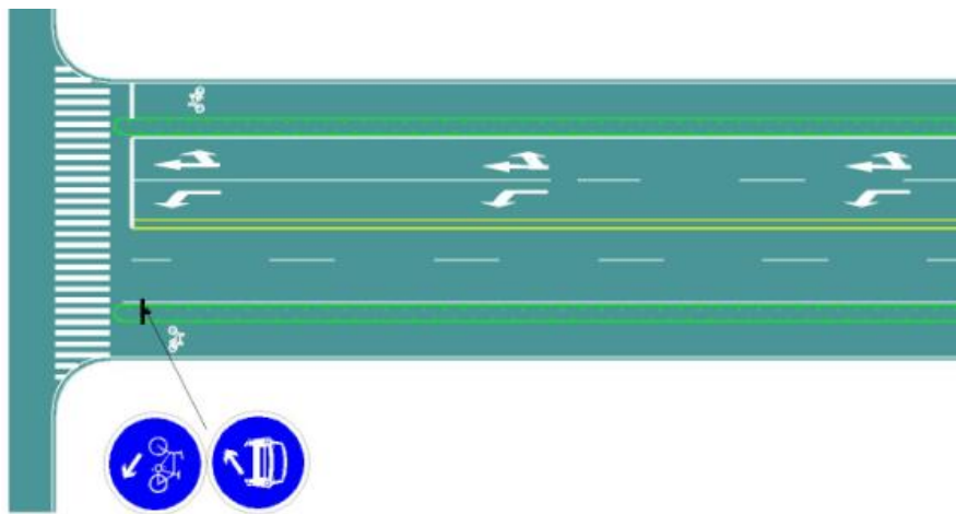
图 118 采用分隔带隔离机非分道标志标线协调设置示例
