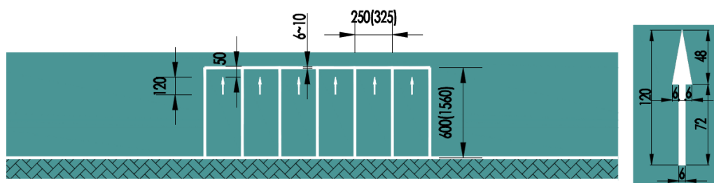
图 12.12.8 固定停车方向停车位标线设置示例 单位：cm
