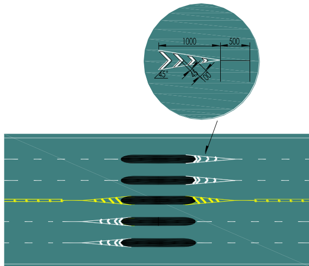
图 14.3.5 收费岛路面标线设置示例 单位: cm
