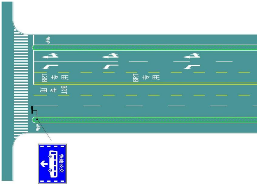
图 123 BRT 专用道标志标线协调设置示例
