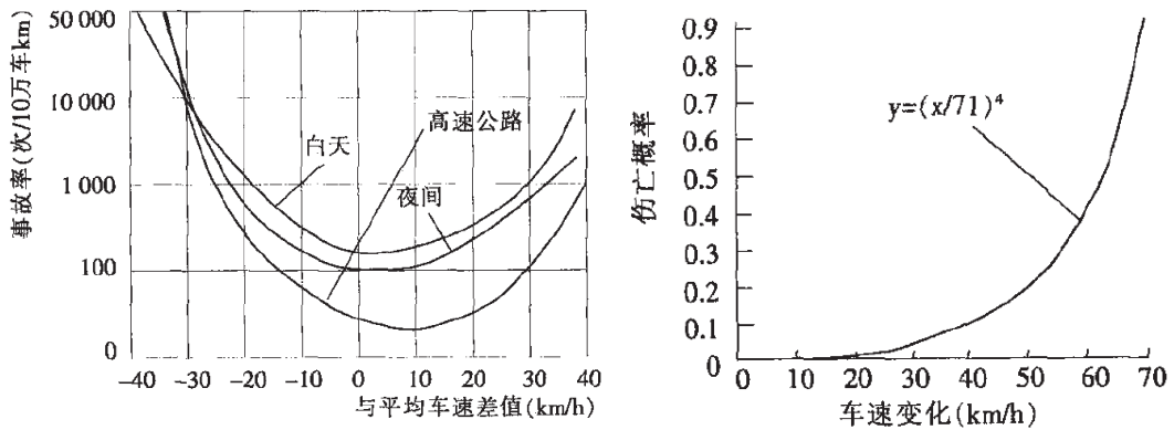
图 34 车辆运行速度与行人死亡或事故率的关系
