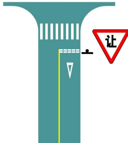
图 109 减速让行标志标线协调设置示例
