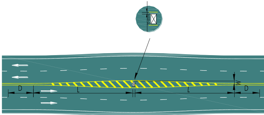
图 14.3.4-1 接近道路中心障碍物标线设置示例 单位: cm
