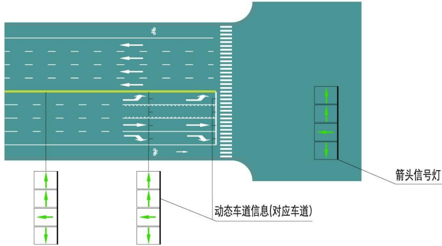
图 85 可变导向车道线设置示例
