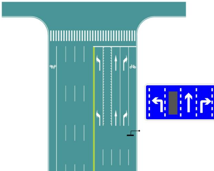
图 105 可变车道标志标线协调设置示例
