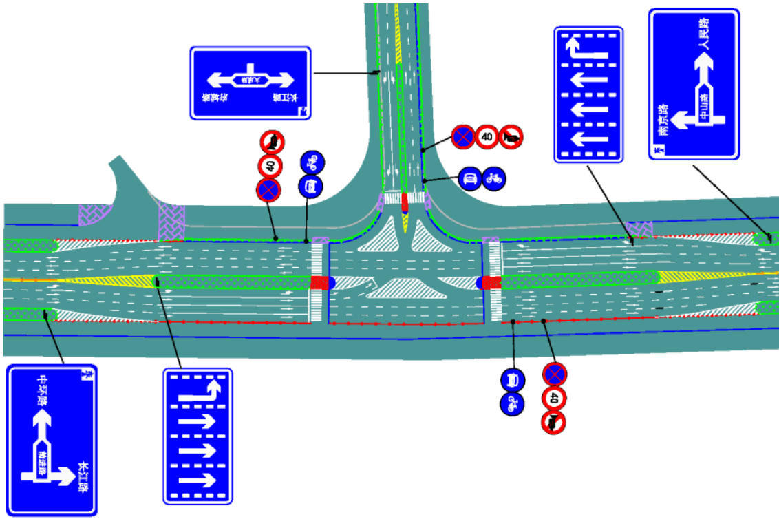
图 106 T 型交叉口示例
