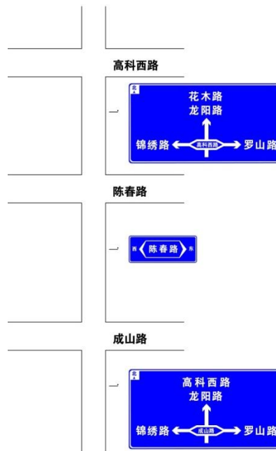
图 60 插入第 III 类告知标志时信息连续的设置
