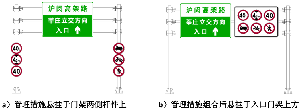
图 69 入口标志组合管理措施
