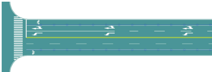
图 119 采用活动式护栏隔离机非分道标志标线协调设置示例
