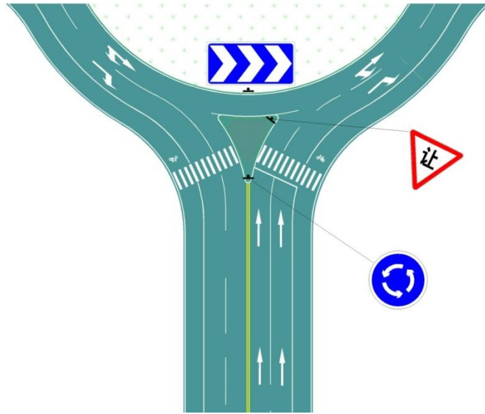
图 111 非灯控环岛标志标线协调设置示例
