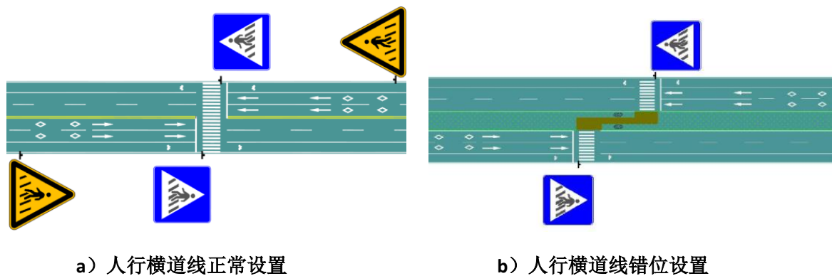
图 116 路段非灯控人行横道标志标线协调设置示例
