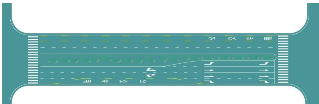
图 96 公交专用车道线设置示例 (2)
