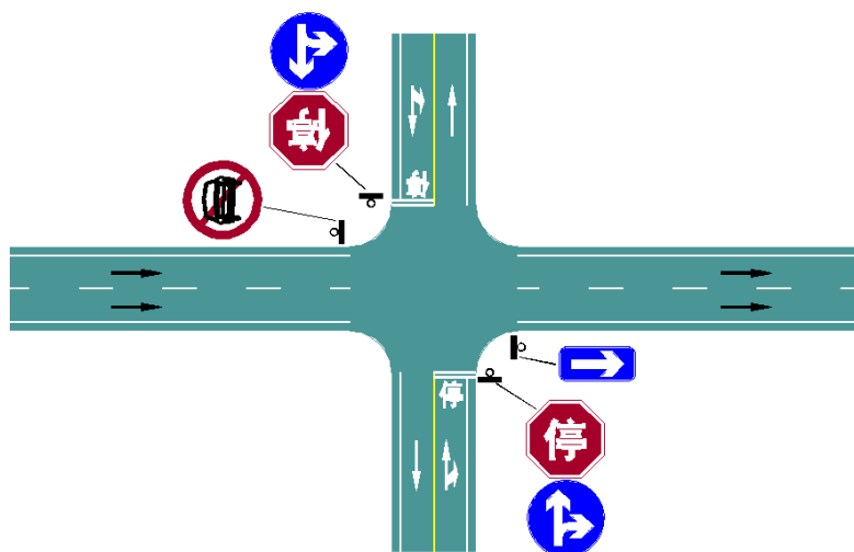
图 21 非灯控单行路交叉口标志的设置
