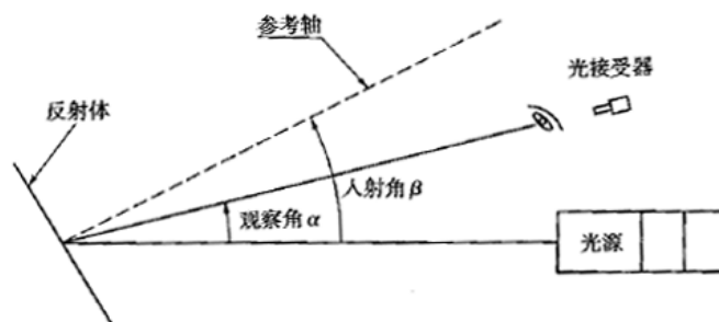
图 100 反射体与灯光、驾驶员视线的关系
