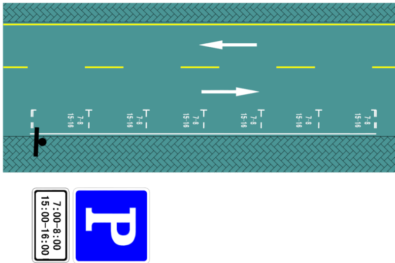
图 130 限时停车位标志标线协调设置示例
