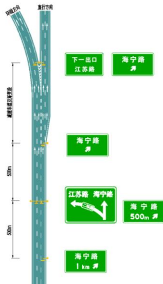
图 74 快速环线转向交通作主线指引的设置
