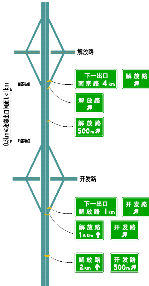
图 78 进出口间距在 0.5km~1km 出口指引标志的设置
