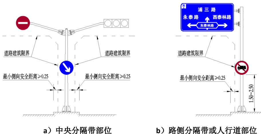
图 13 标志及支撑结构边缘距车行道路面边缘的最小侧向安全距离
