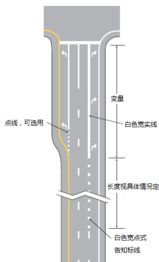
图 89 车道变换告知标线设置
