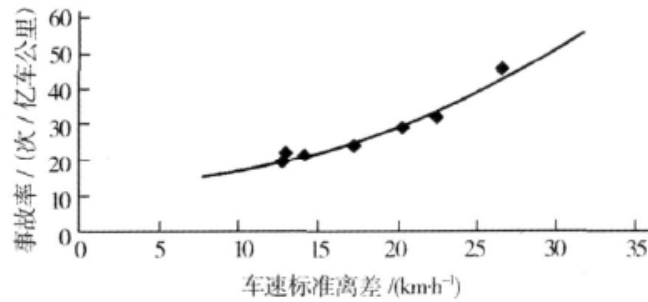
图 35 车速标准差与事故率关系图
