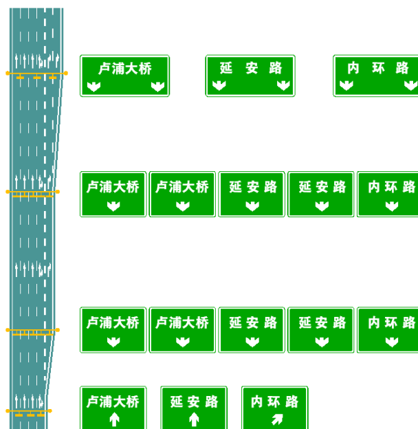
图 81 连续分合流路段指路标志的设置
