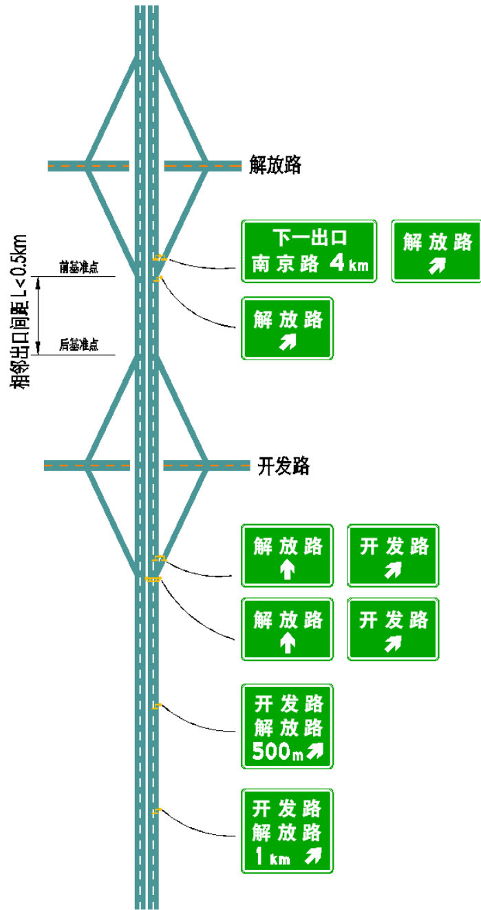
图 79 进出口间距小于 0.5km 出口指引标志的设置一
