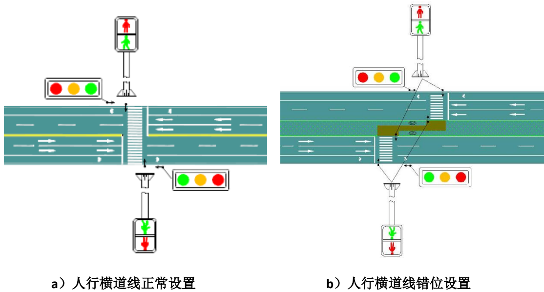
图 117 路段灯控人行横道标志标线协调设置示例
