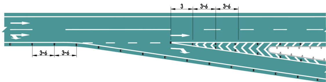
图 99 出口匝道突起路标布设例 单位：cm
