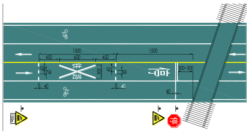
图 14.4.3 无人看守的铁路平交道口标线设置示例 单位：cm
