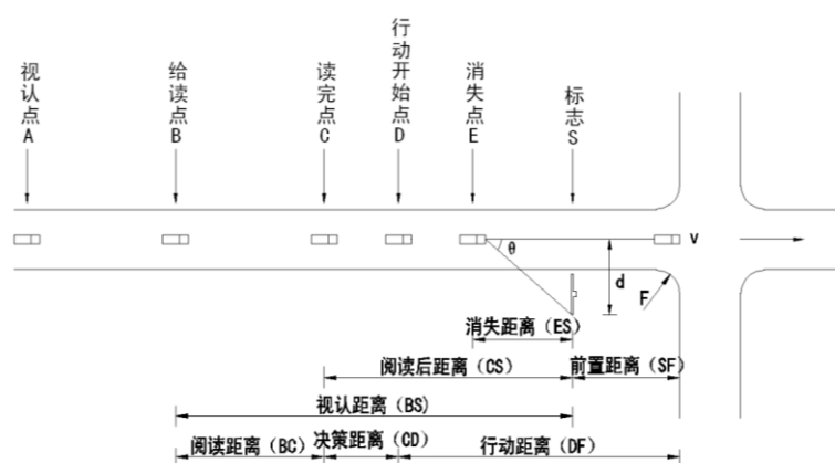
图 8 标志的识读过程
