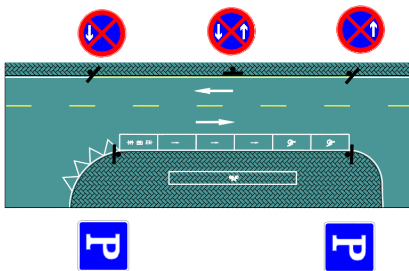
图 129 停车位标志标线协调设置示例
