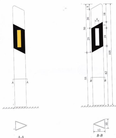
图 101 柱式轮廓标
