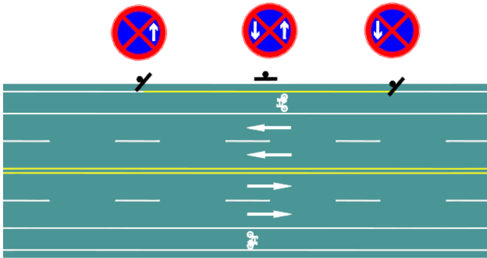
图 135 禁止停车标志标线协调设置示例一
