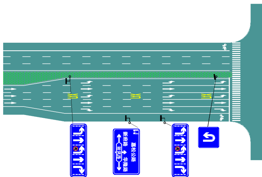
图 23 渠化车道多级变化交通流量较大时分向行驶车道标志的设置
