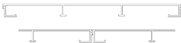
图 18 小尺寸板材挤压成型拼接
