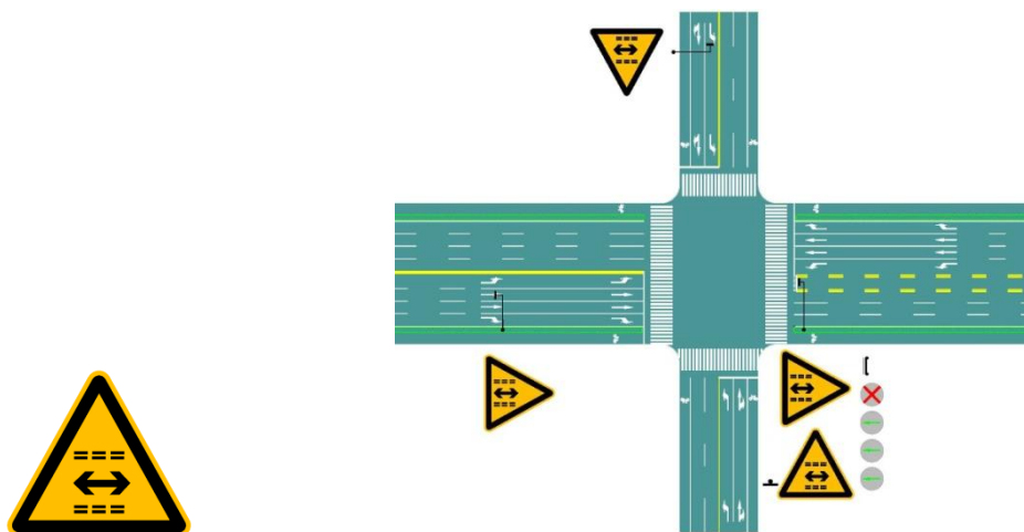
图 44 注意横向道路潮汐车道标志
