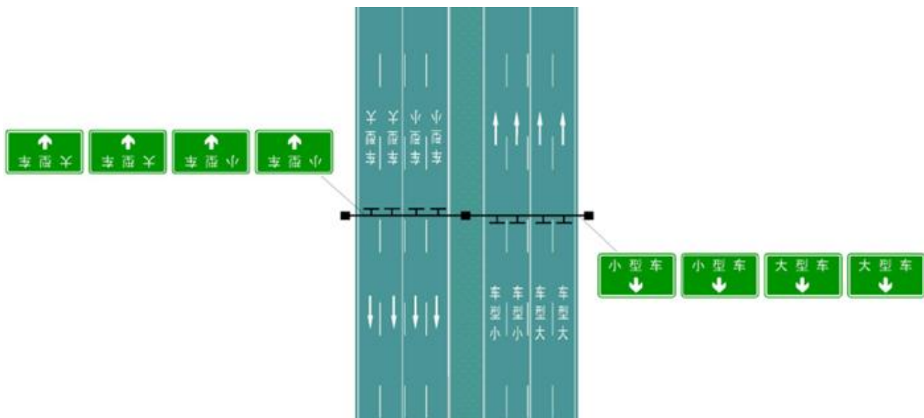
图 125 大小型车分车道行驶标志标线协调设置示例
