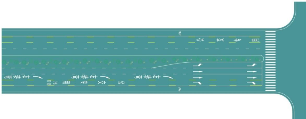
图 95 公交专用车道线设置示例 (1)
