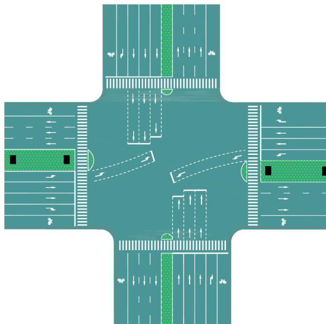
图 12.6.2 待行区线设置示例 单位：cm
