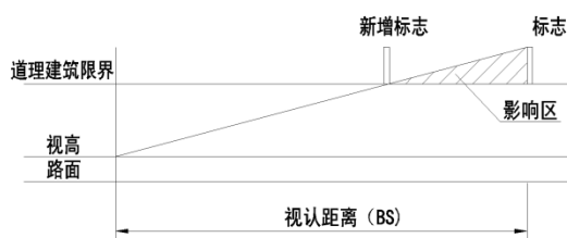
图 10 道路上方标志
