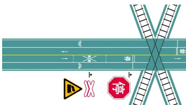
图 41 两股或两股以上的无人看守铁路道口标志设置
