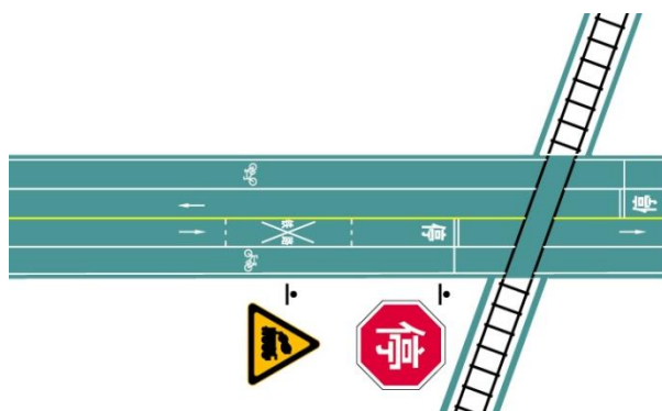
图 39 无人看守铁路道口标志与标线配合
