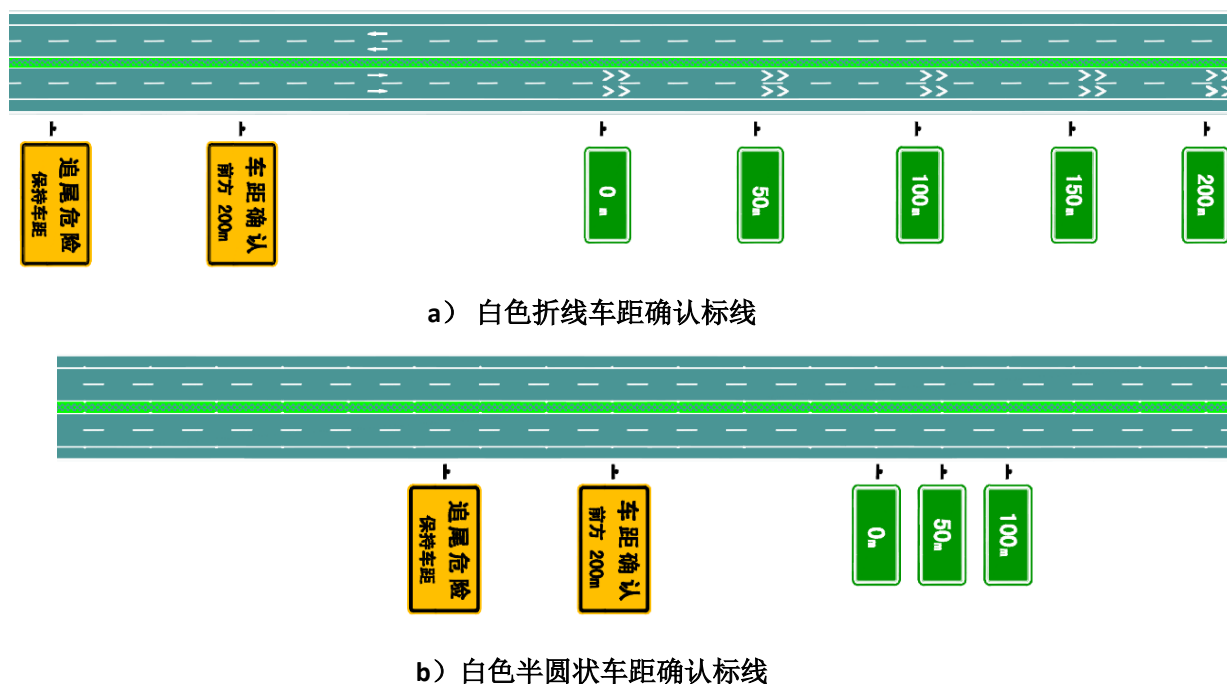
图 128 车距确认标志标线协调设置示例
