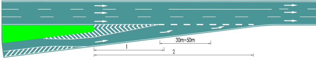
图 12.11.3-1 道路入口标线设置示例 单位: cm 1-三角地带标线长度与纵向标线的实线段长度之和 2-入口段总长
