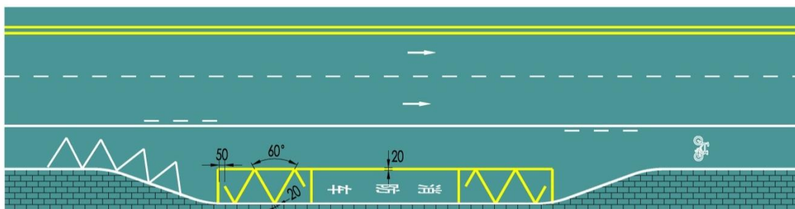
图 93 非机动车道边缘专用车辆港湾式停靠站设置示例 单位: cm
