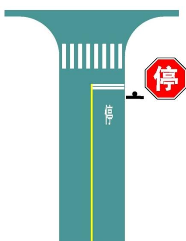
图 108 停车让行标志标线协调设置示例
