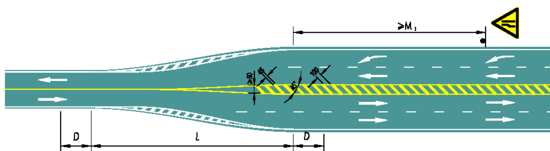
图 13.2.7 单黄实线与双黄实线搭接设置示例 单位：cm
