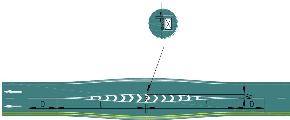
图 14.3.4-1 接近道路中心障碍物标线设置示例 单位: cm
