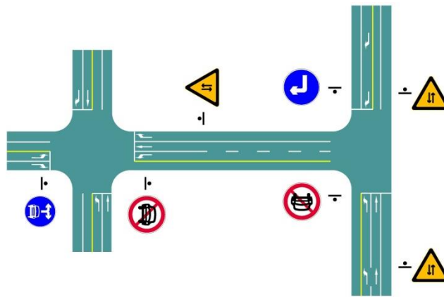
图 42 双向交通标志的设置 1
