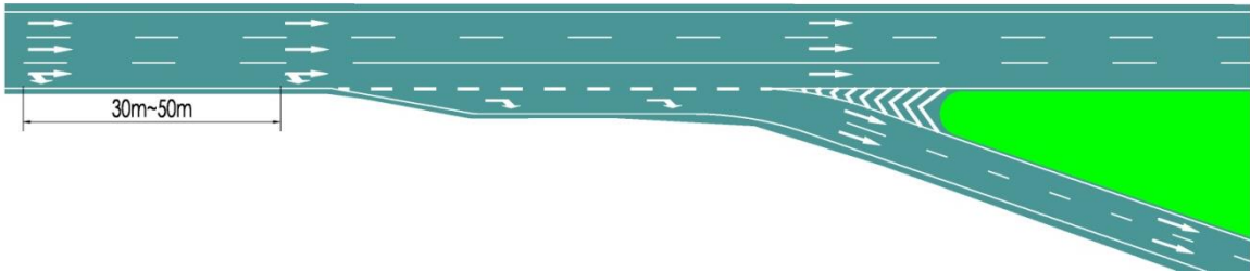
图 12.11.3-2 道路出口标线设置示例
