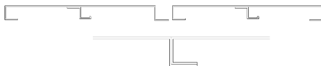
图 17 小尺寸板材经 90° 折弯处理并在板材背部铆接拼接
