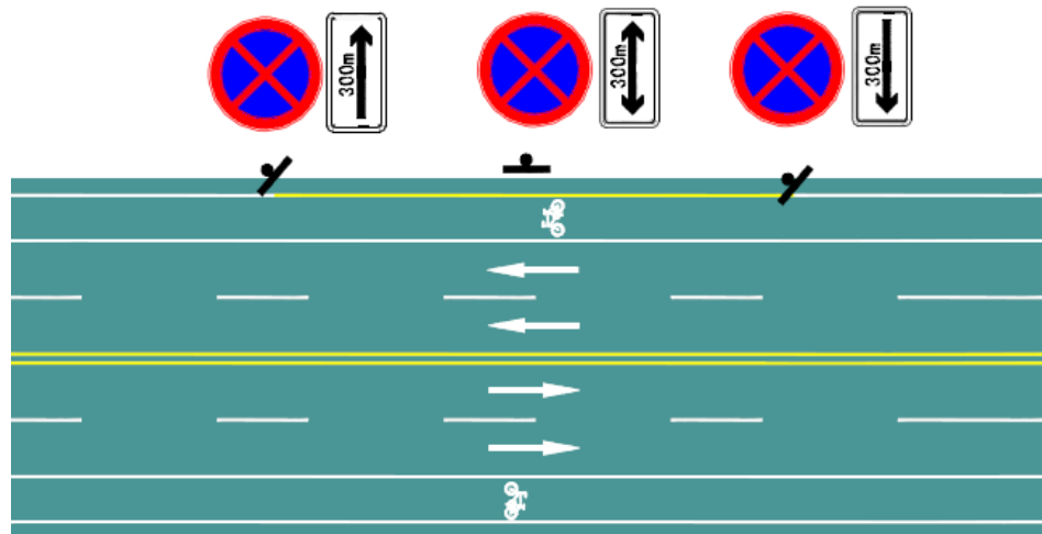
图 136 禁止停车标志标线协调设置示例二
