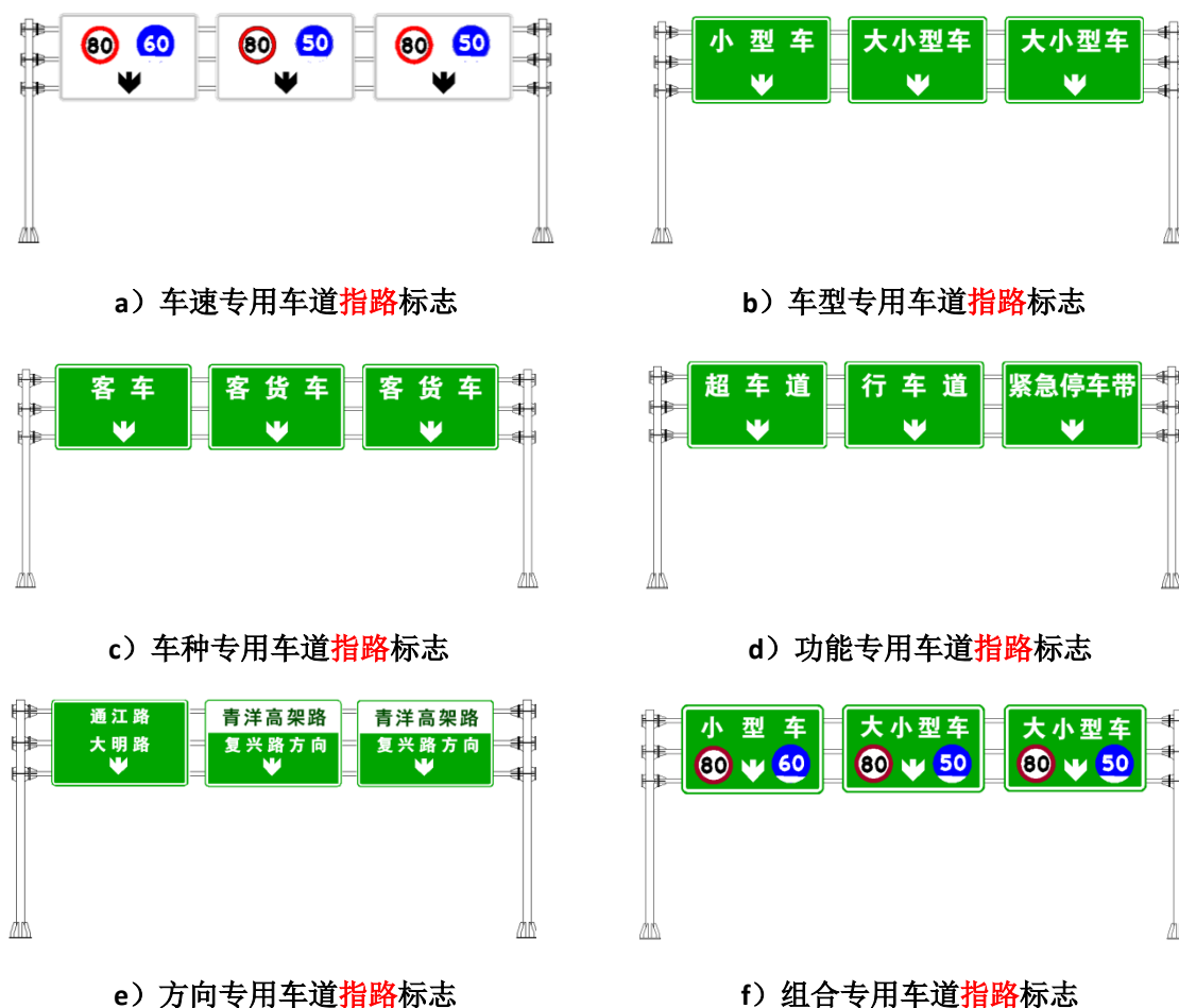
图 73 快速路车道 指路标志
