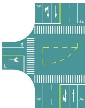
图 13.7.5 T 形交叉路口非机动车禁驶区标线设置示例
