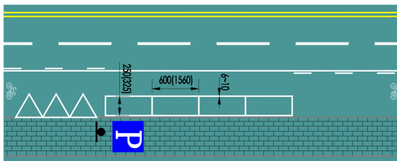
图 90 路边式停车位标线设置示例 单位：cm
