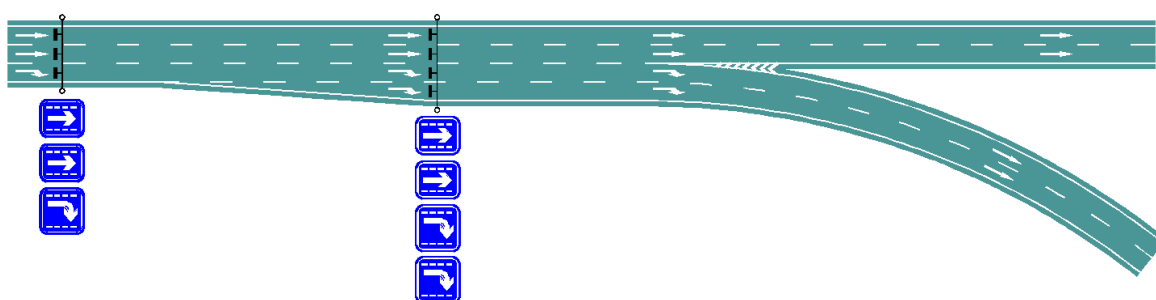
图 24 多车道逐级分流时车道行驶车道标志的设置
