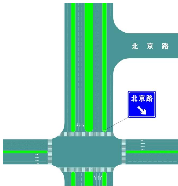
图 62 地点方向标志的设置
