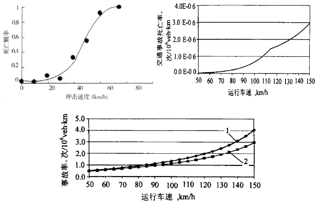
图 34 车辆运行速度与行人死亡或事故率的关系
