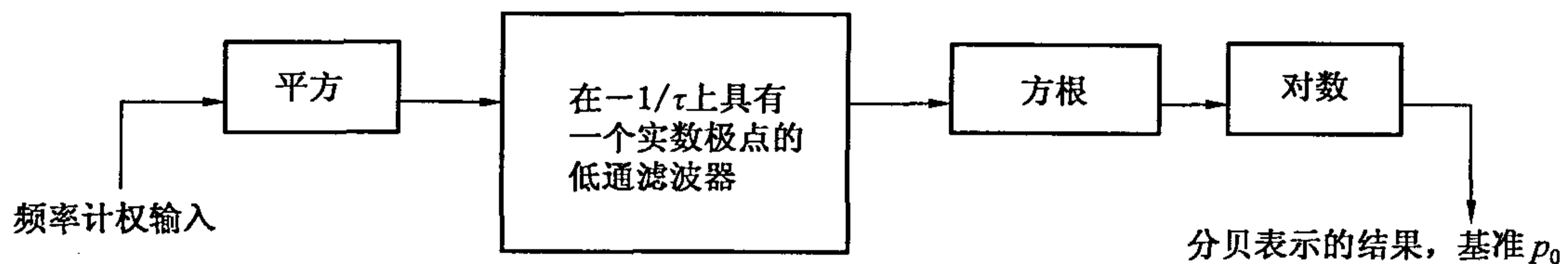
图 1 形成指数时间计权声级的主要步骤
