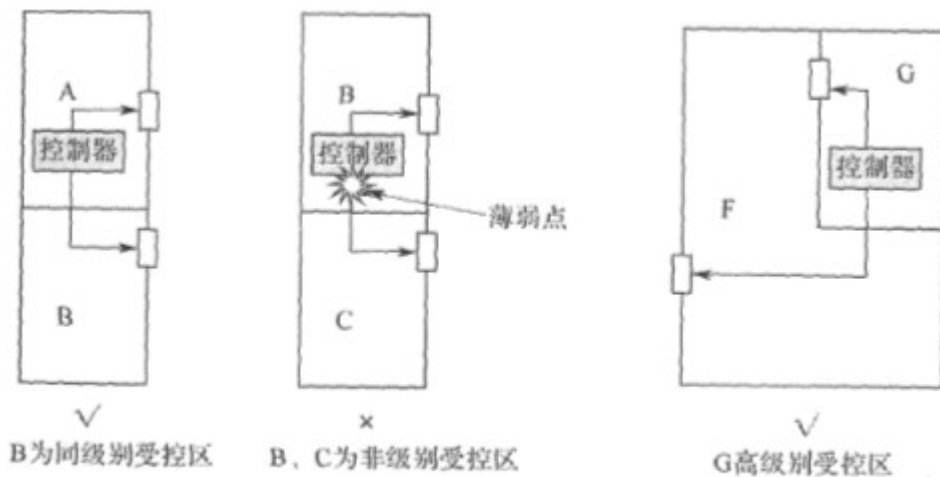
图7 现场设备在不同受控区安装时对安全的影响
