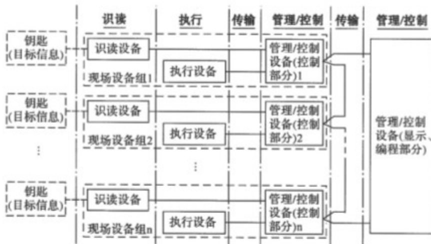
图 4.0.5-2 环线制系统组成
