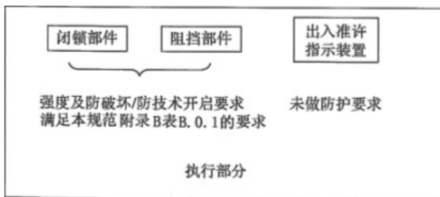
图 3 对执行部分的防护要求
