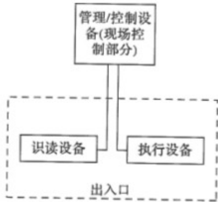
图 4.0.4-1 单出入口控制设备型组成
