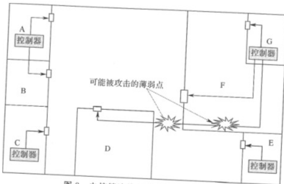
图8 电控锁连线的布设对安全的影响
