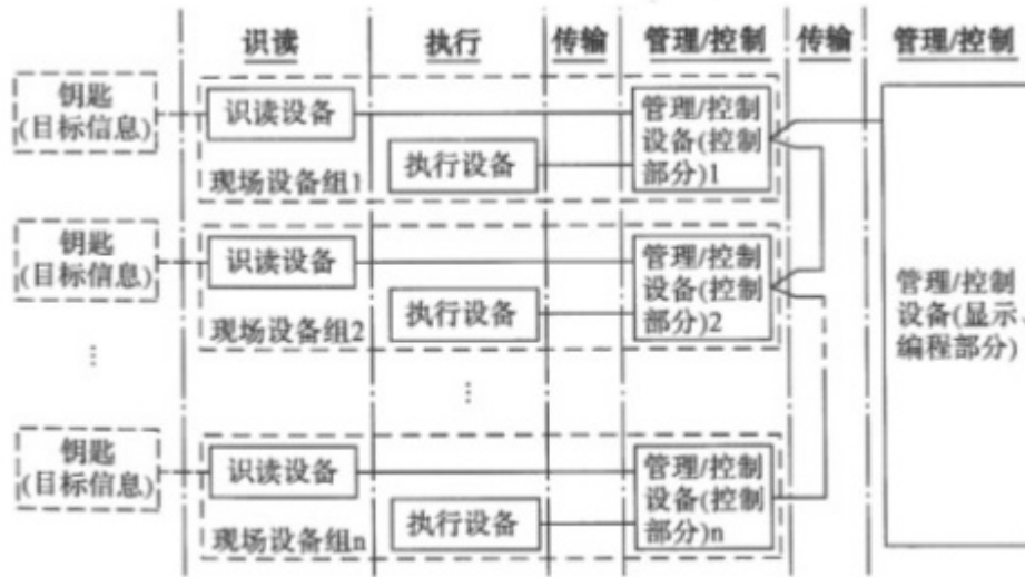
图 4.0.5-1 总线制系统组成
