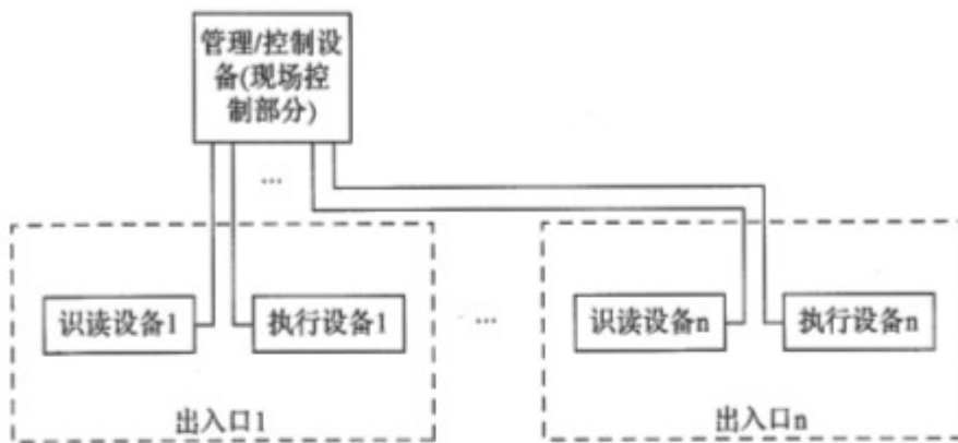
图 4.0.4-2 多出入口控制设备型组成
