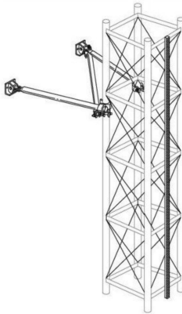
图 3 典型的附着架
