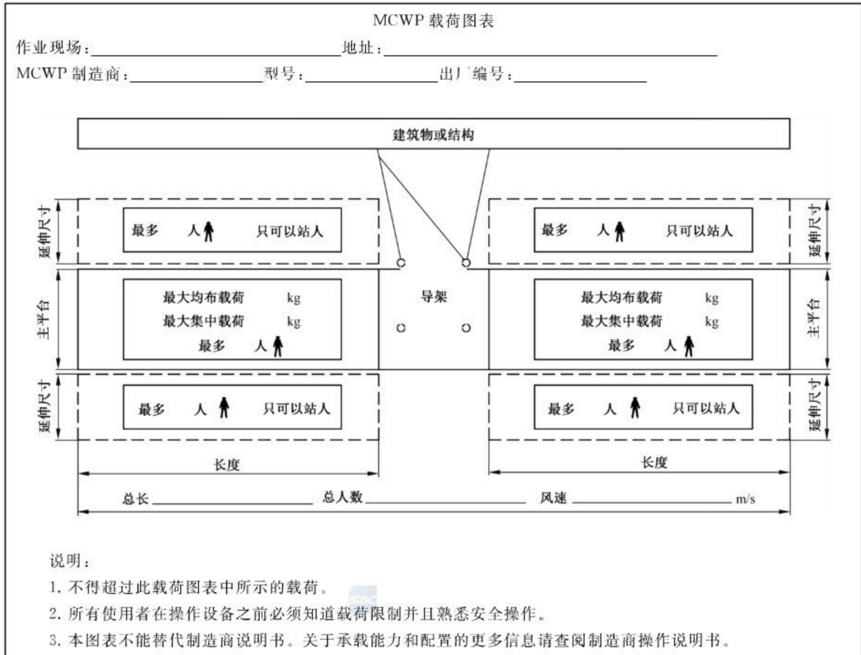
图 4 载荷图例
