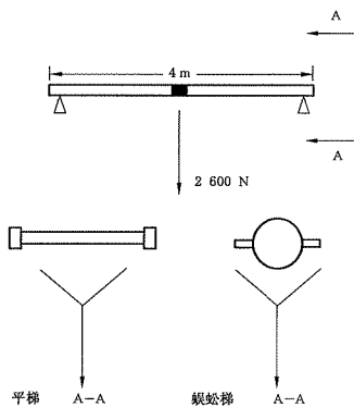
图 B.1 水平强度试验布置图
