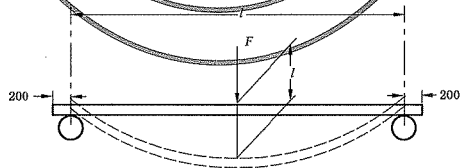
图 B.5 水平弯曲试验
