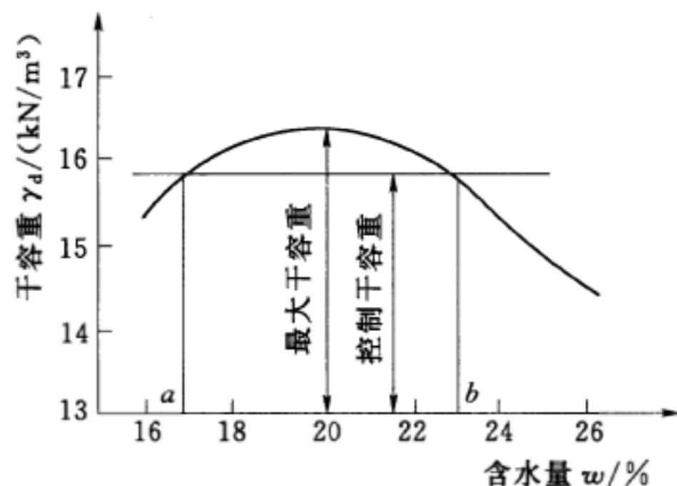
图8 黏性土击实试验曲线
