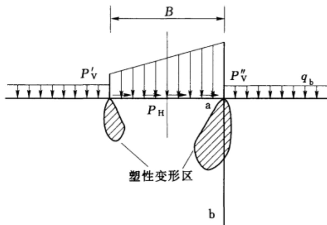
图 H. 0. 2 塑性变形区示意图
