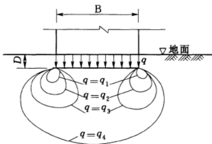
图3 塑性变形区变化示意图
