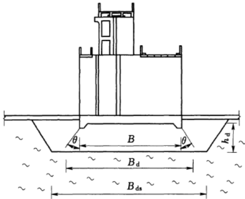
图7 换土(砂)垫层示意图
