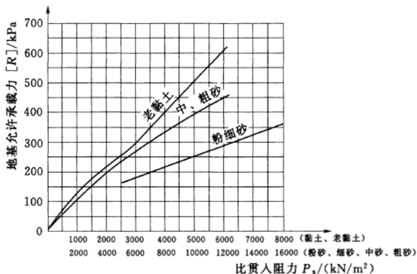
图 5 比贯入阻力与地基允许承载力相关关系
