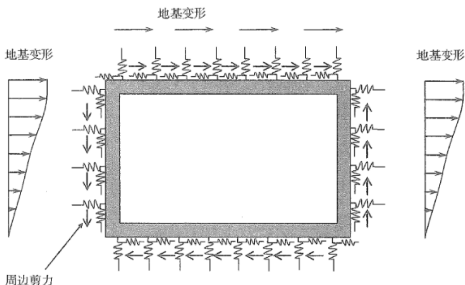
图 2 反应位移法计算模型
