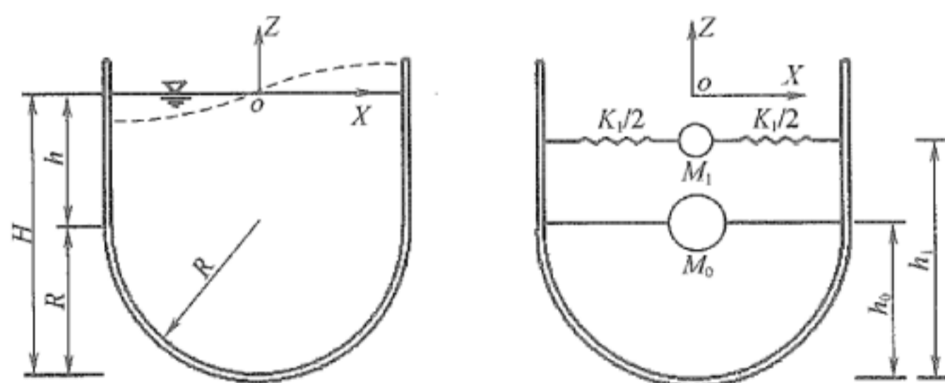
(b) U形渡槽
