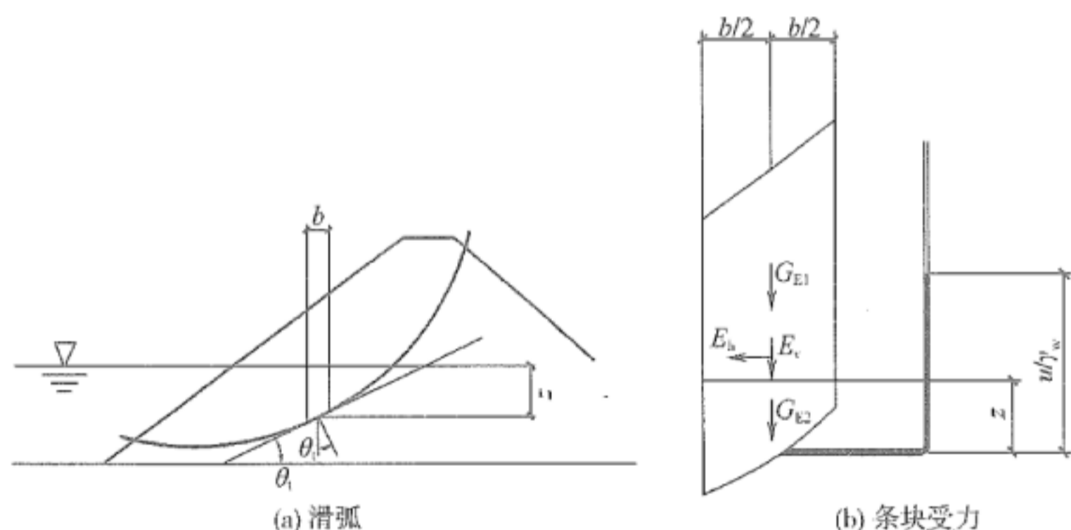
图 A.0.1 滑弧和条块受力示意图
