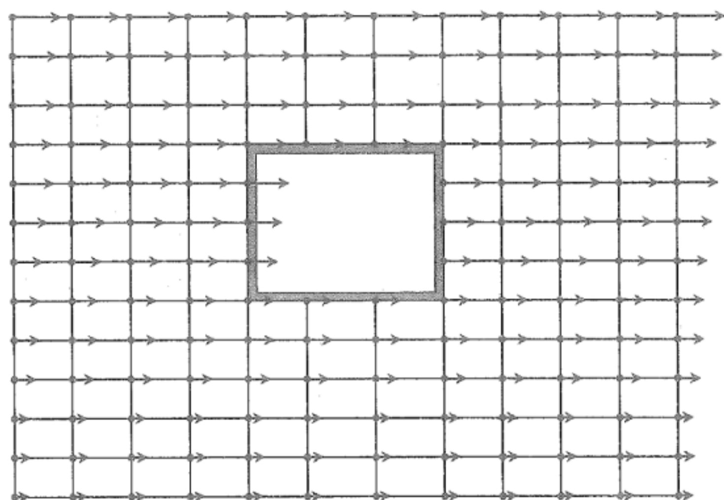
图3 有限元反应加速度法计算模型
