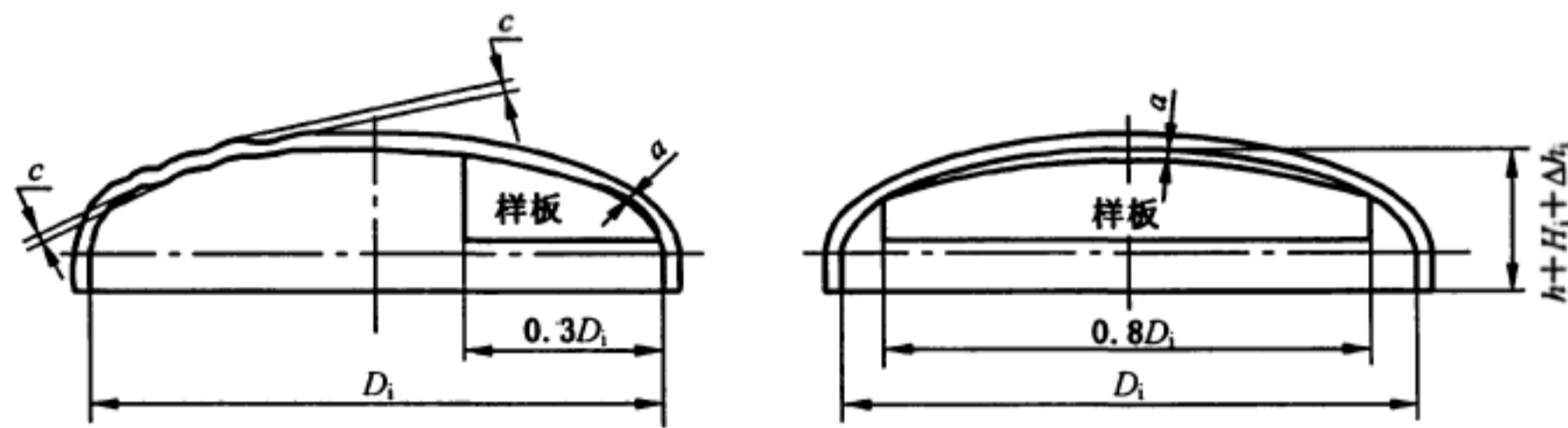
图 4 封头形状尺寸公差示意图
