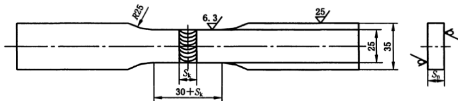
图 8 拉伸试样加工尺寸
