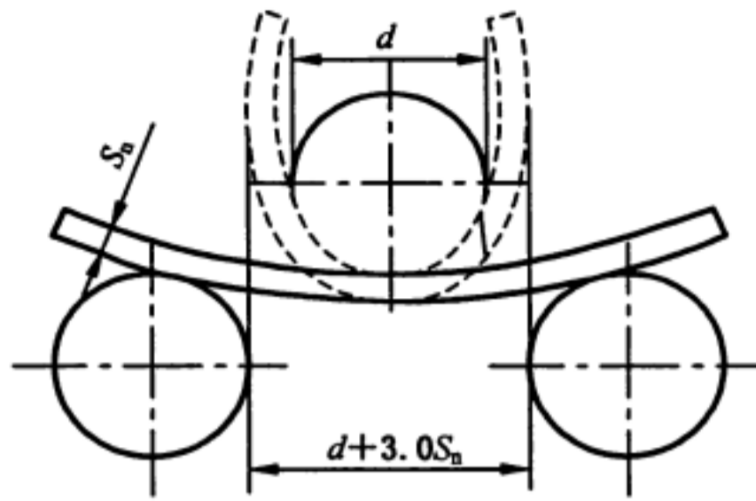
图9 弯曲试验示意图
