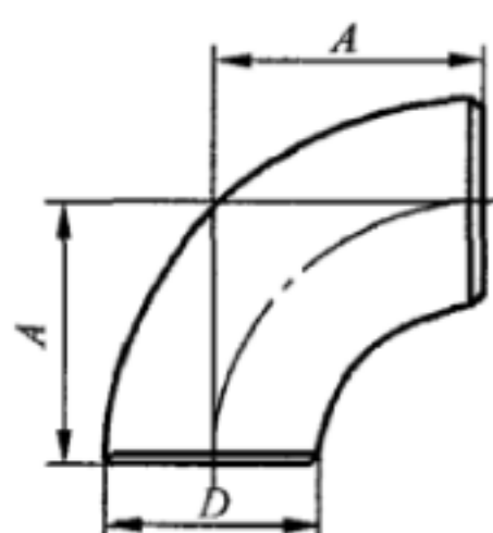
图 4 短半径 90°弯头
