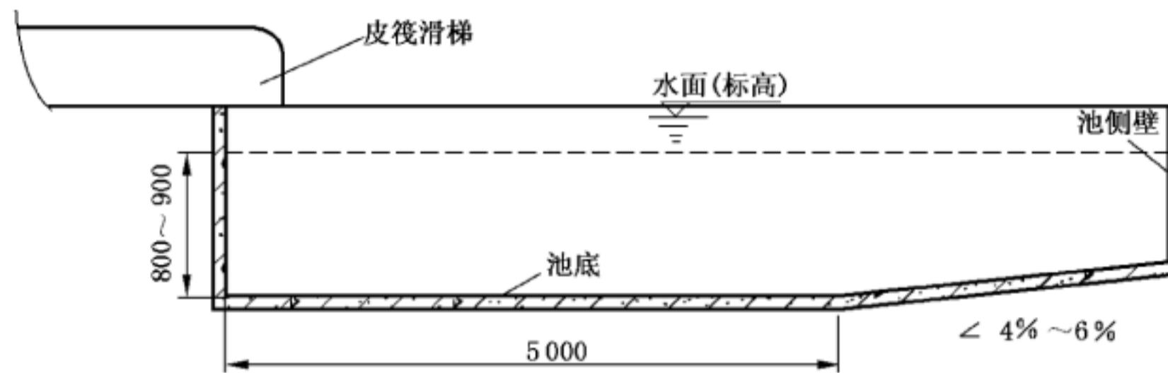
图3 皮筏滑梯末端及溅落区相关尺寸
