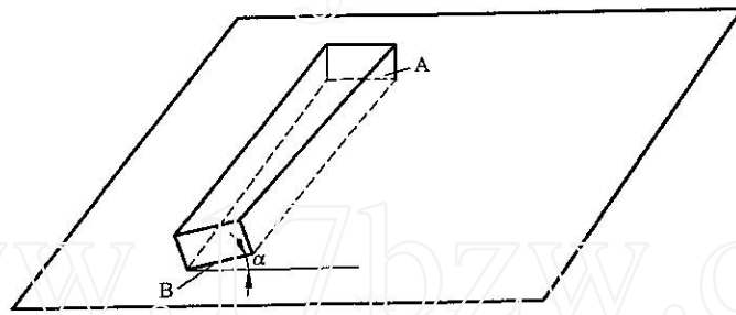
图 A.1 扭拧度测量示意图
