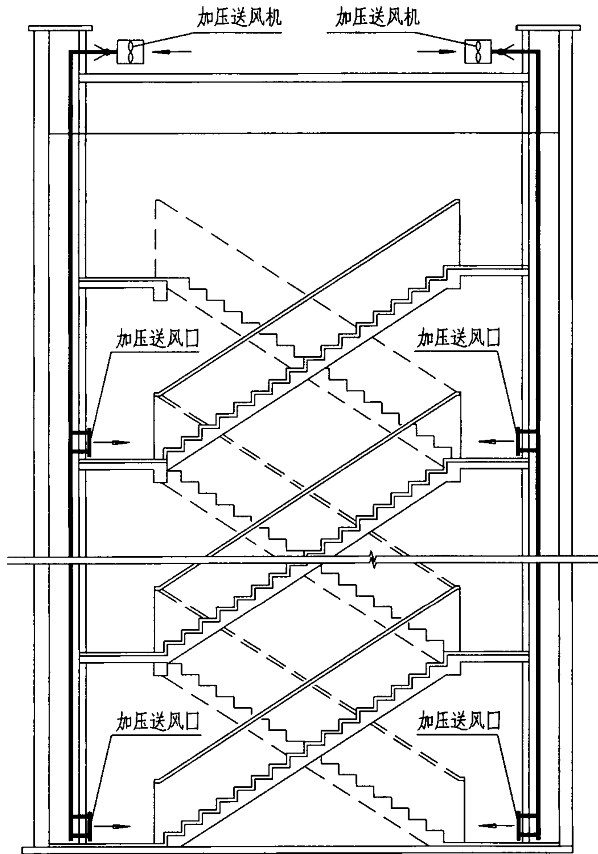
A-A剖面图
