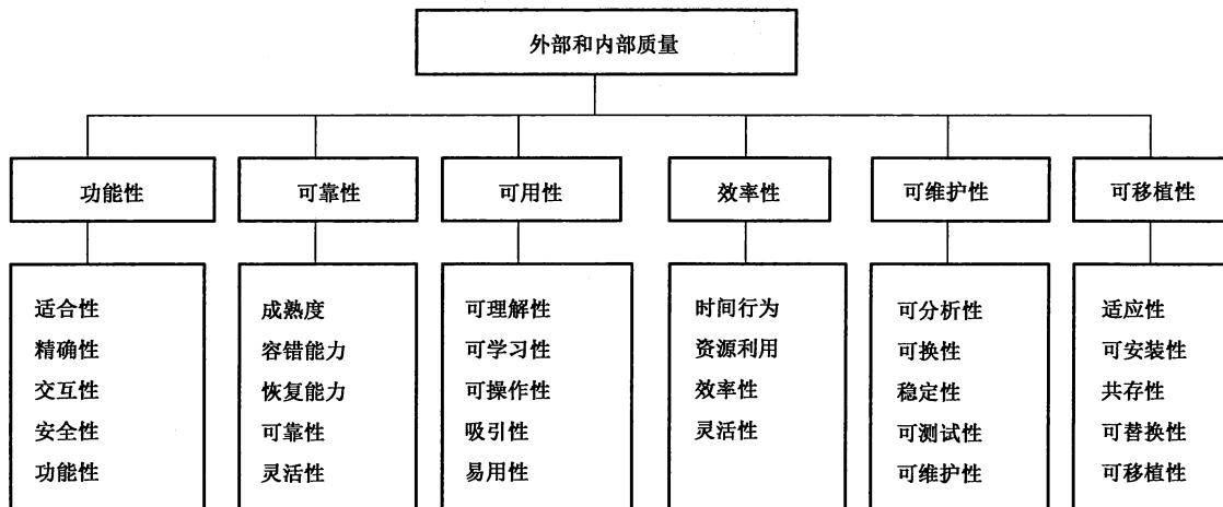
图 2 质量模型的外部 and 内部特征,描述特征和子特征
