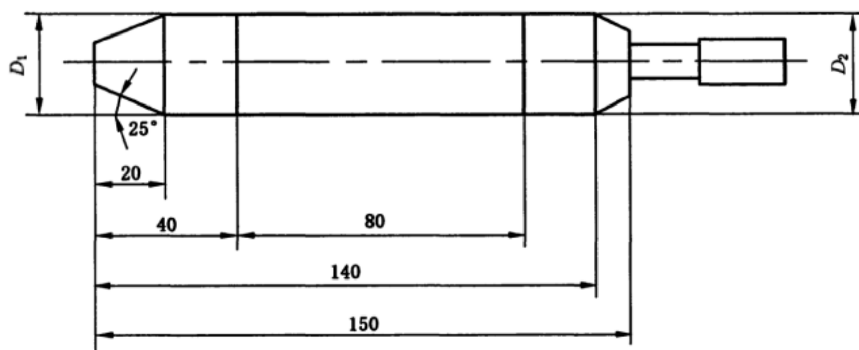
图1 塞规
