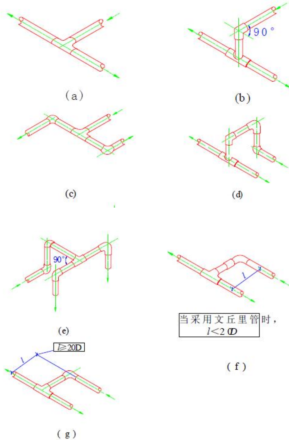
图 B 管网分支结构图
