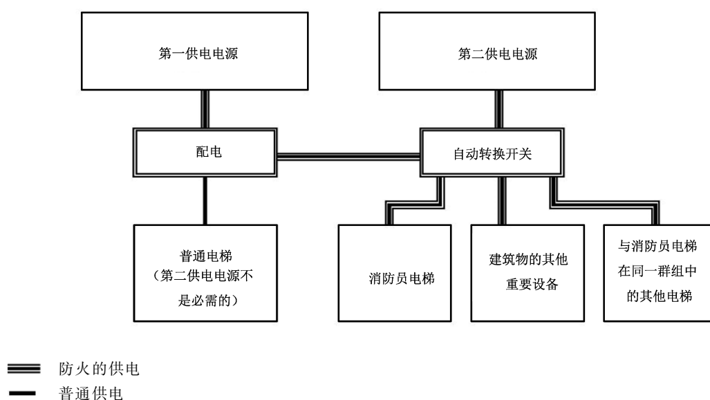
图 B.1 消防员电梯供电电源示例
