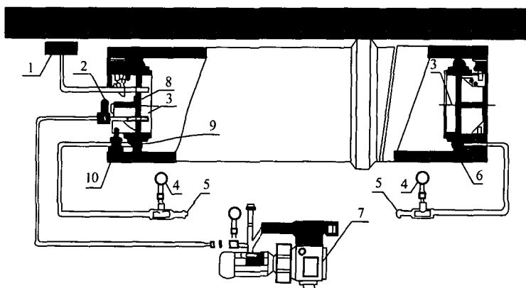
图 E.0.1 排水管道闭气检验装置图
