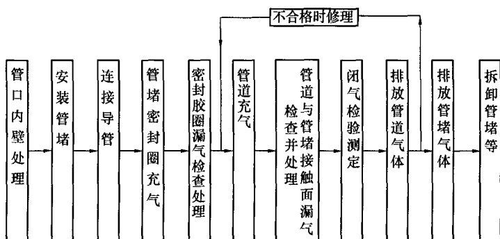
图 E.0.2 管道闭气检验工艺流程图
