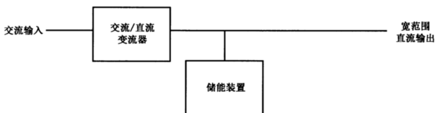
图 B.1 储能装置直接连接至输出
