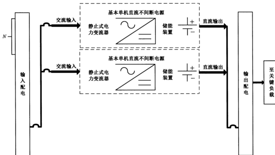
图 A.2 按负载大小配置的无冗余系统( N 个直流不间断电源单元)
