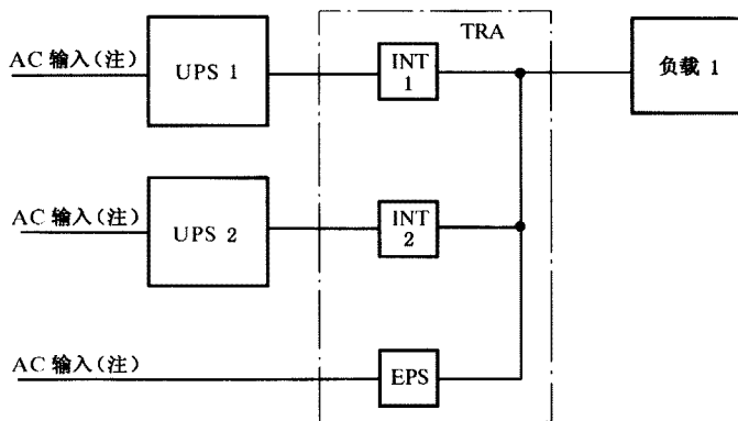
图 C.11 多功能开关
