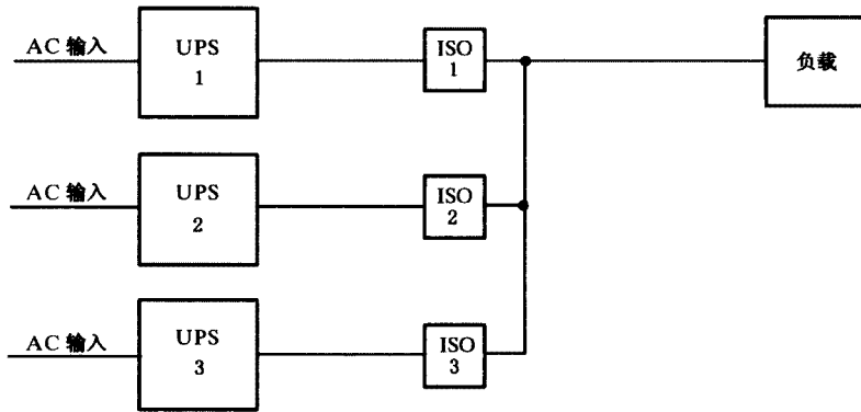
图 C.8 用于 UPS 断路器的隔离开关
