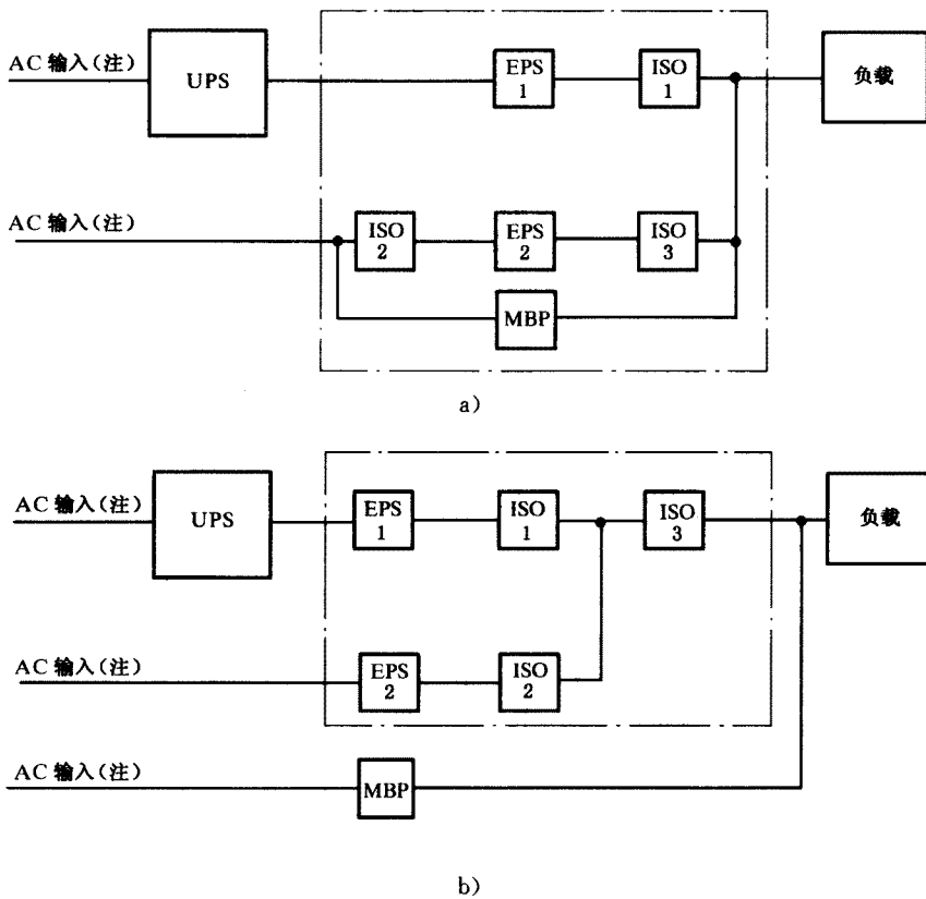
图 C.9 维修旁路开关
