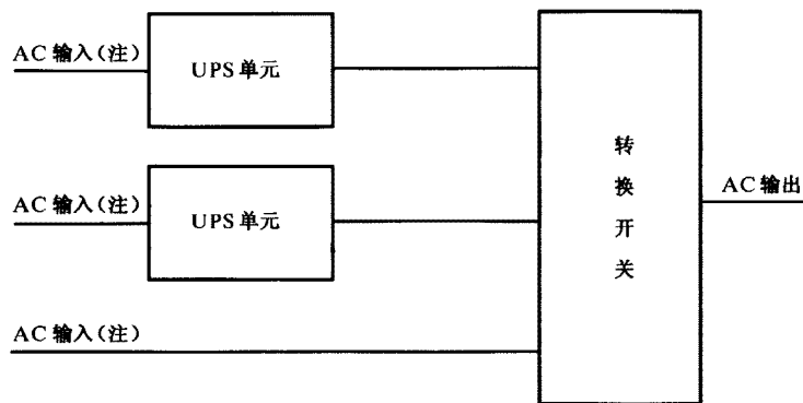
图 A.7 带旁路的备用冗余 UPS
