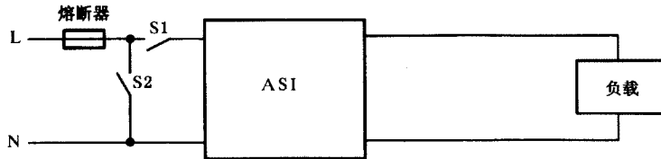
图 G.1 试验电路的连接
