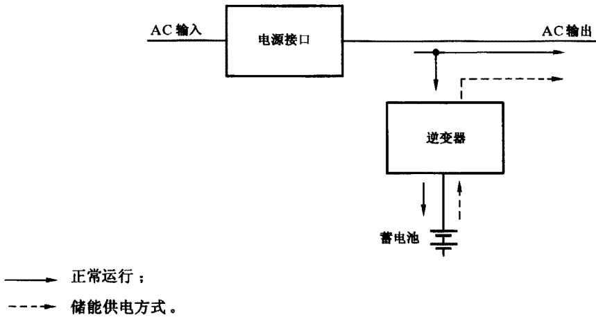
图 B.3 UPS 互动运行
