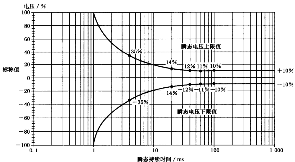
图 2 二类动态输出性能
