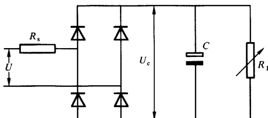
图 E.1 基准非线性负载
