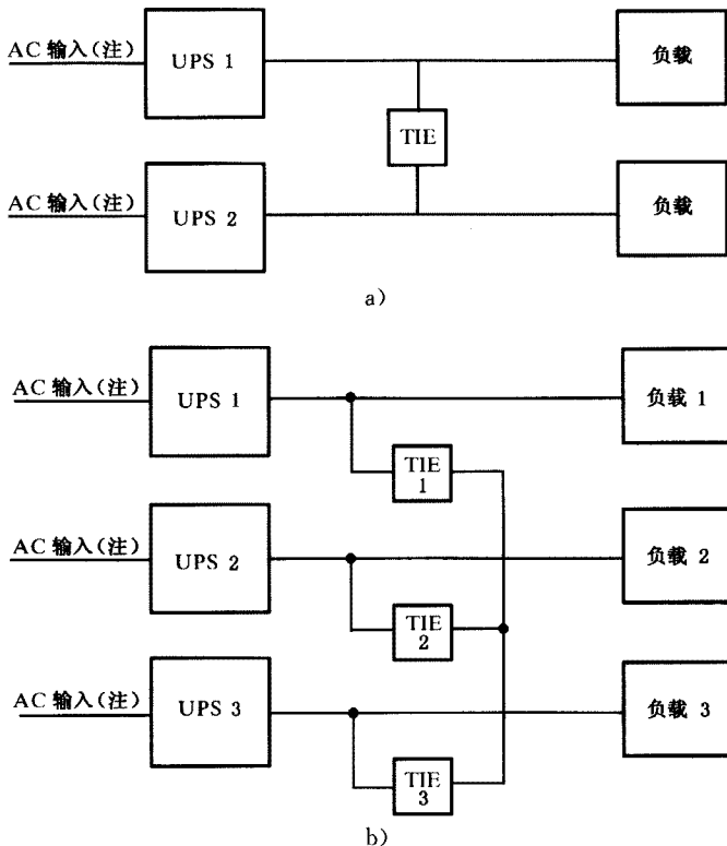
图 C.10 互连开关
