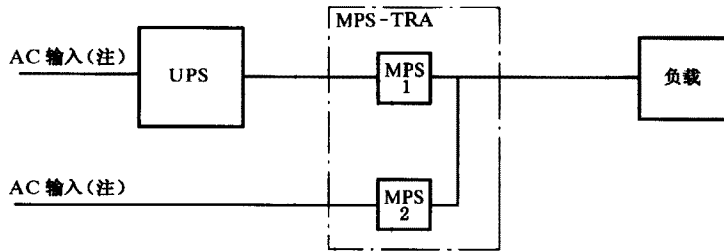
图 C.2 机械转换开关
