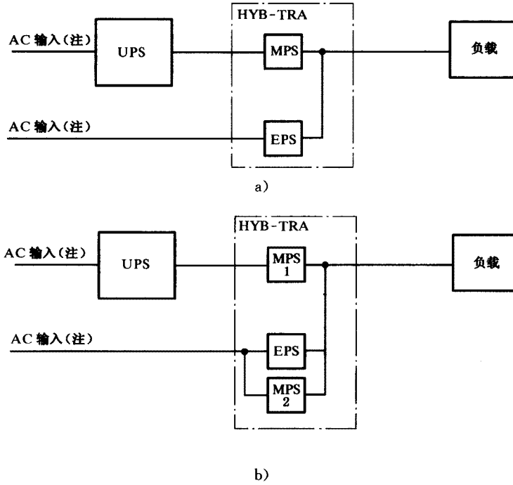
图 C.4 混合转换开关
