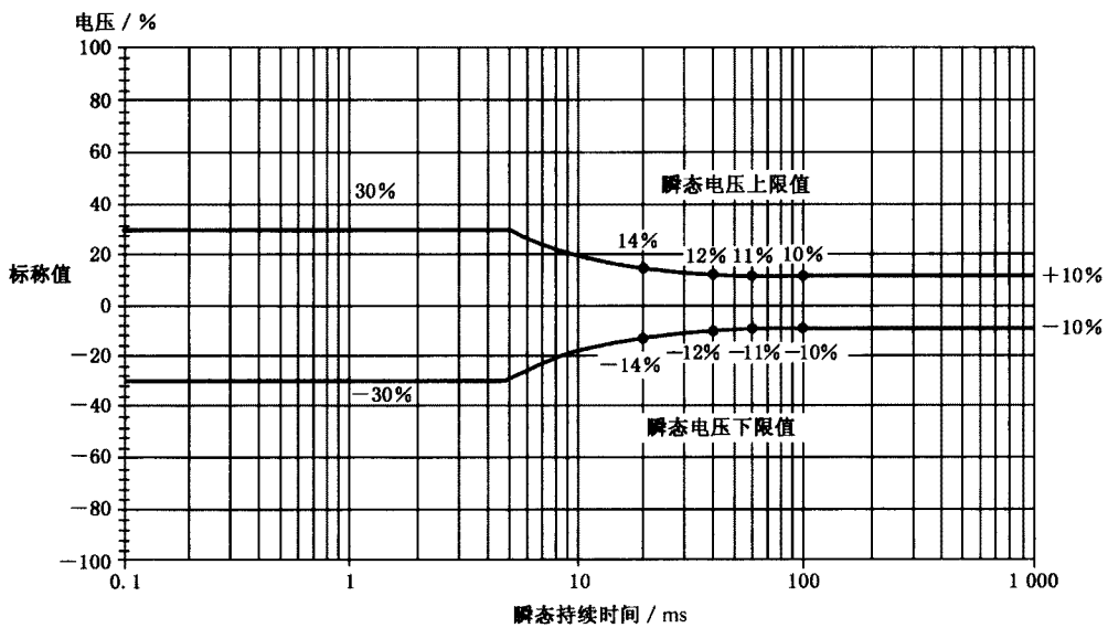
图 1 一类动态输出性能
