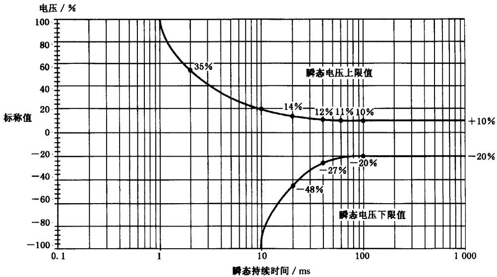
图 3 三类动态输出性能
