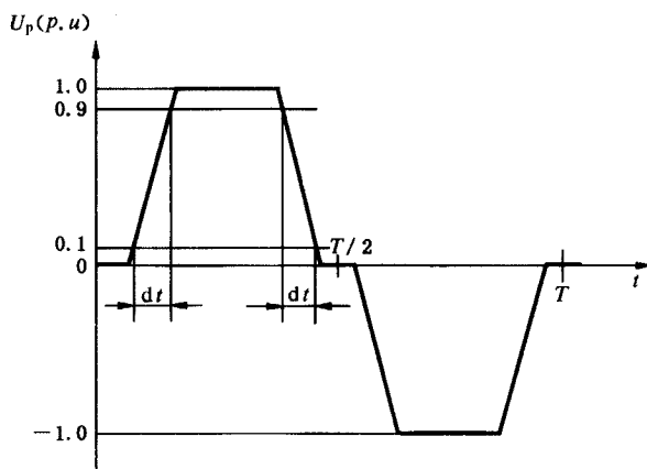
图 4 非正弦输出电压波形的例子
