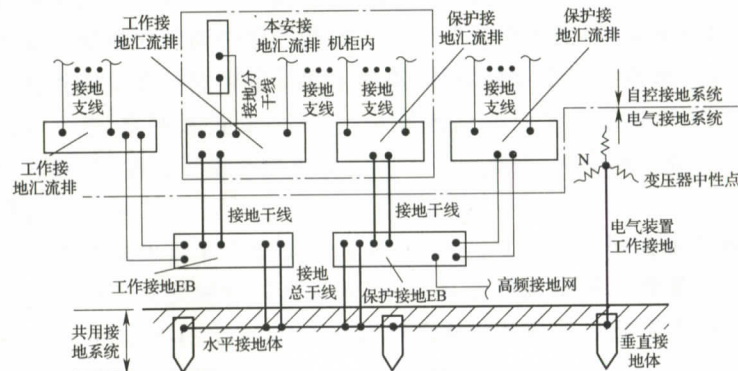
图 3 控制室接地系统示意图
