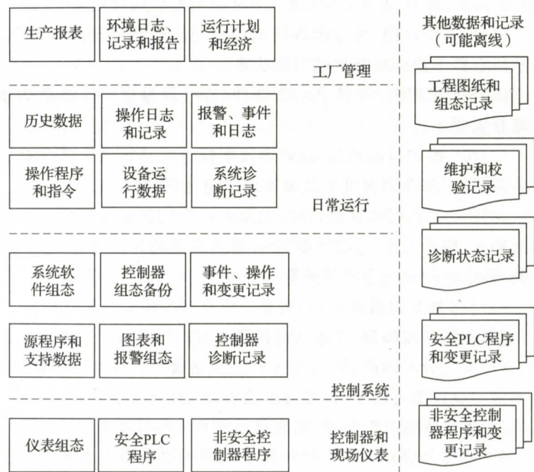
图 2 计算机控制系统数据文件文档结构图
