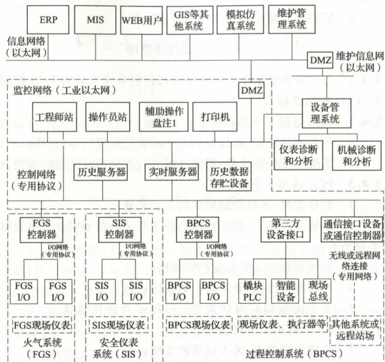
图 3.2.1 典型计算机控制系统结构示意图
