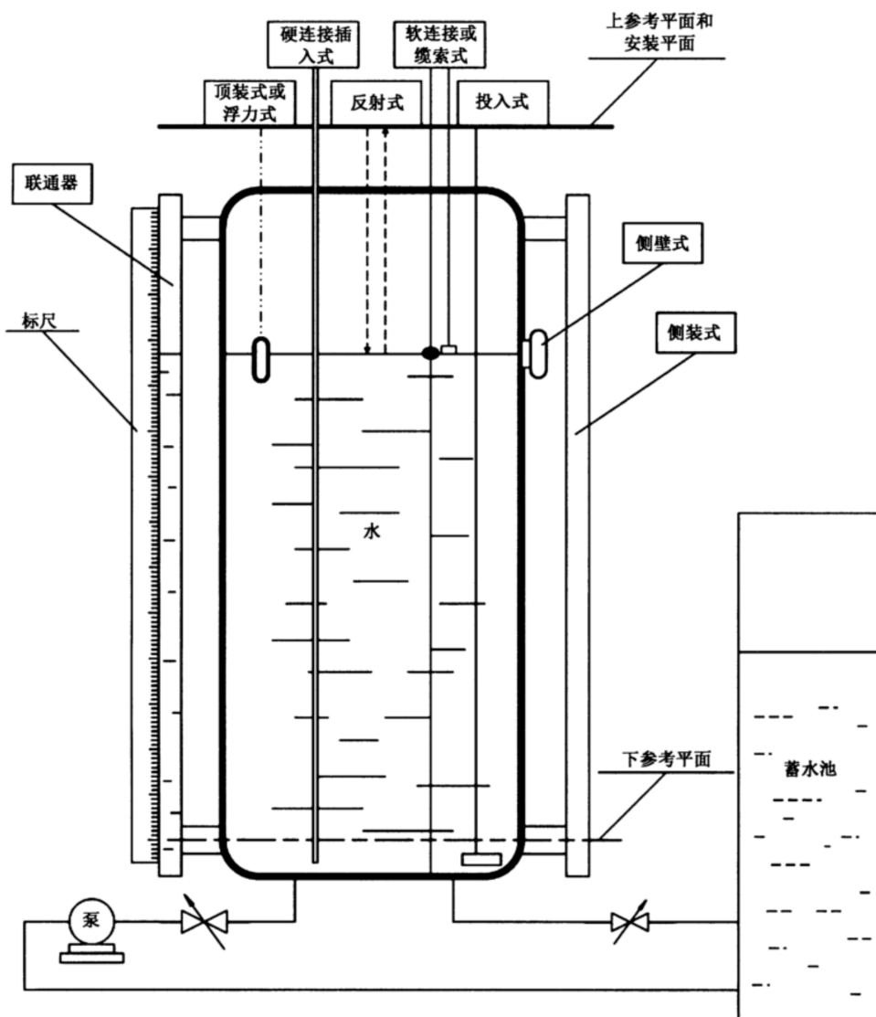
图 2 立式液位检定安装示意图
