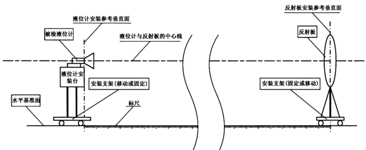
图 1 横式液位模拟检定安装示意图
