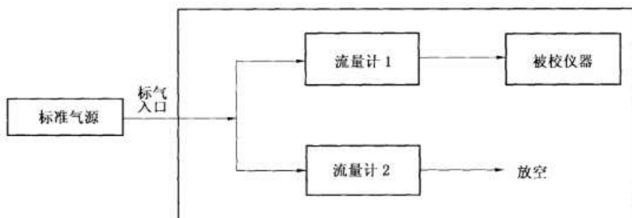
图1 流量控制器示意图
