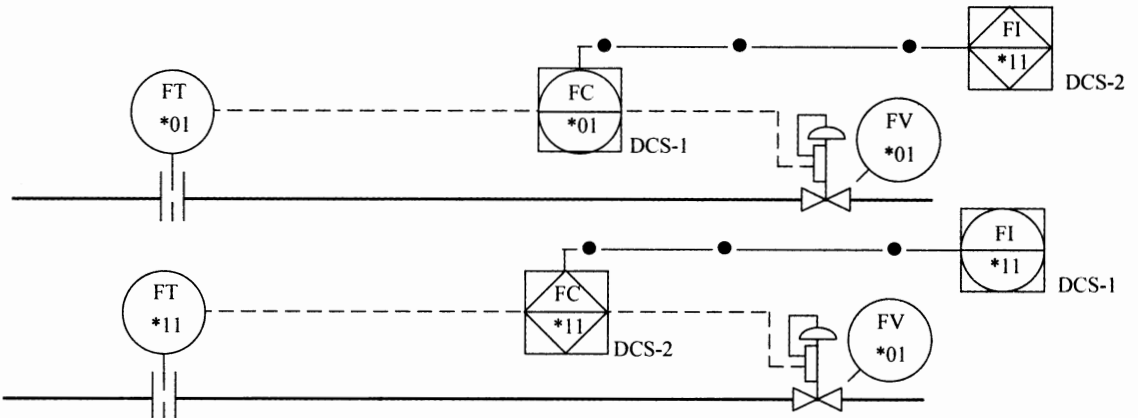
(g) 多种信号线组合(共享显示、共享控制系统—首选和备选系统,电子仪表)
