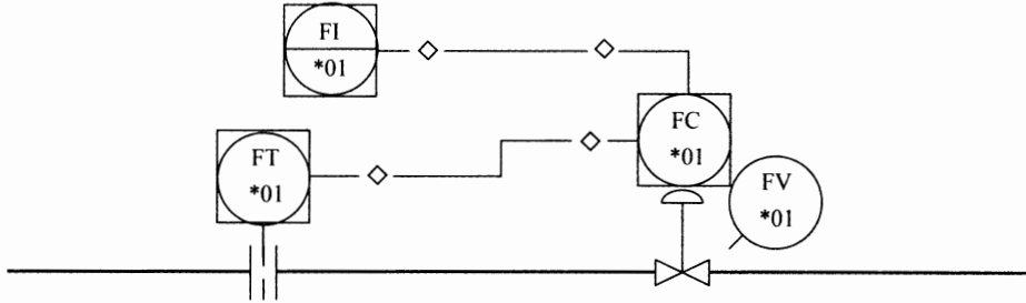
(f) 多种信号线组合(共享显示、共享控制系统,现场总线仪表,电子仪表)
