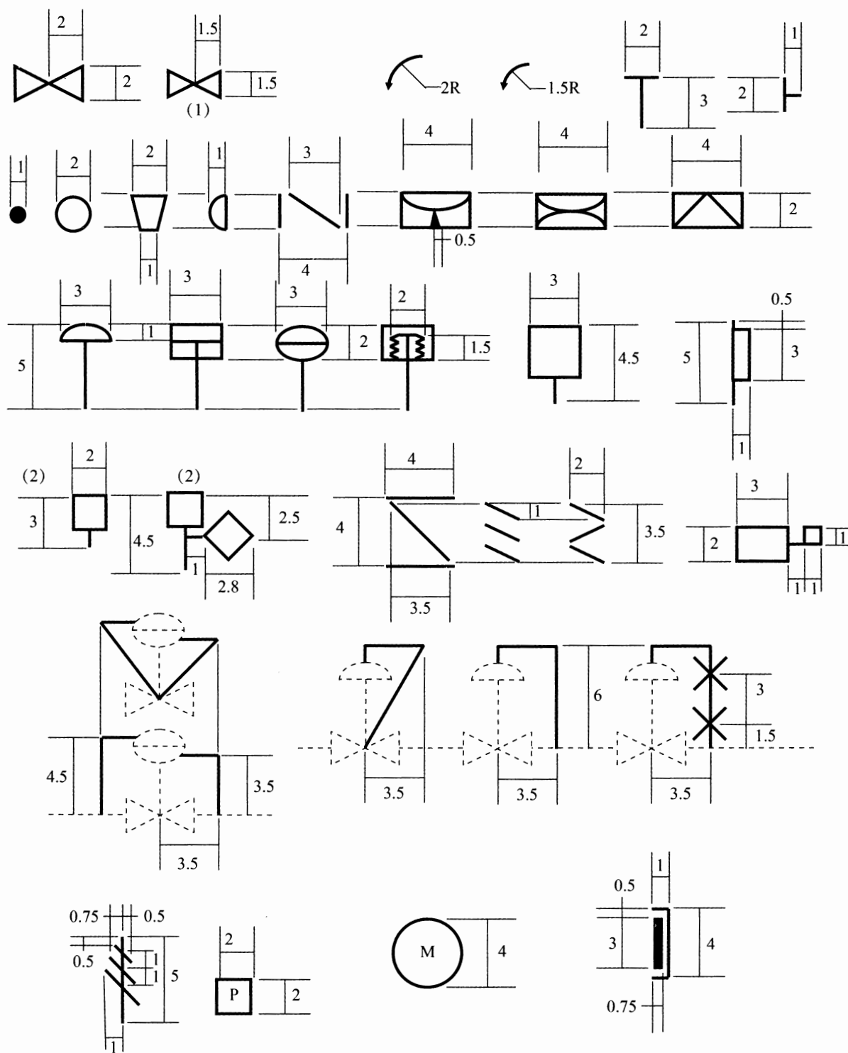
图 5.8.5 表 5.4.1、表 5.4.2、表 5.4.3 和表 5.4.4 图形符号主要比例关系
