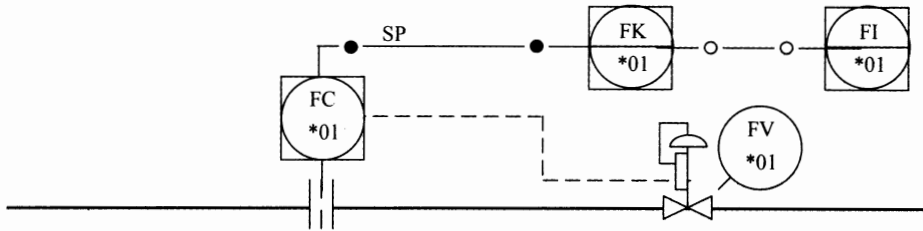
(f) 多种信号线组合(共享显示、共享控制系统,现场总线仪表,电子仪表)
