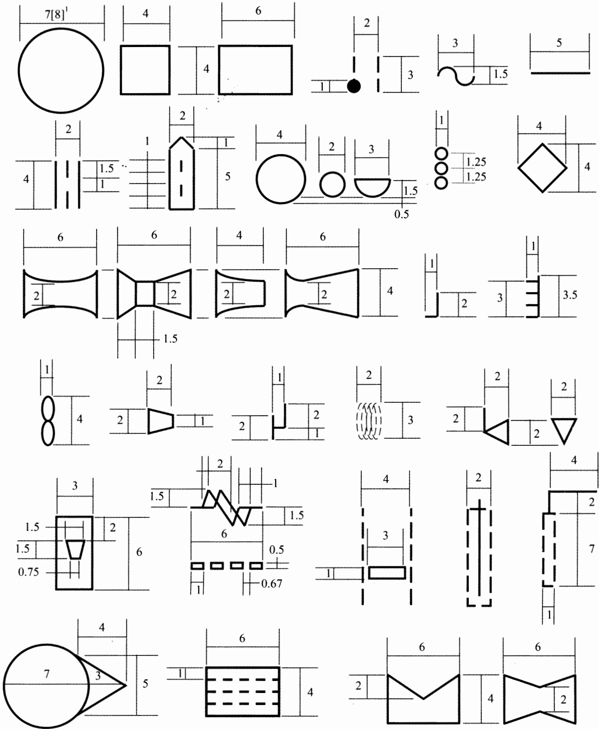
图 5.8.4 表 5.2.1、表 5.2.3、表 5.2.4 和表 5.2.5 图形符号主要比例关系
