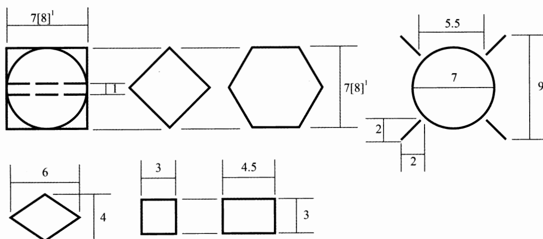
图 5.8.3 本标准第 5.1.1 条和表 5.1.2 图形符号主要比例关系
