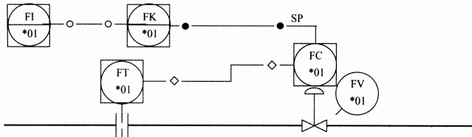
(g) 多种信号线组合(共享显示、共享控制系统—首选和备选系统,电子仪表)
