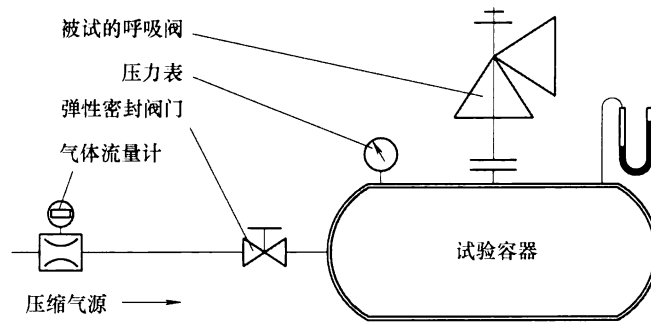
图4 呼吸阀的呼出气量试验系统示意图
