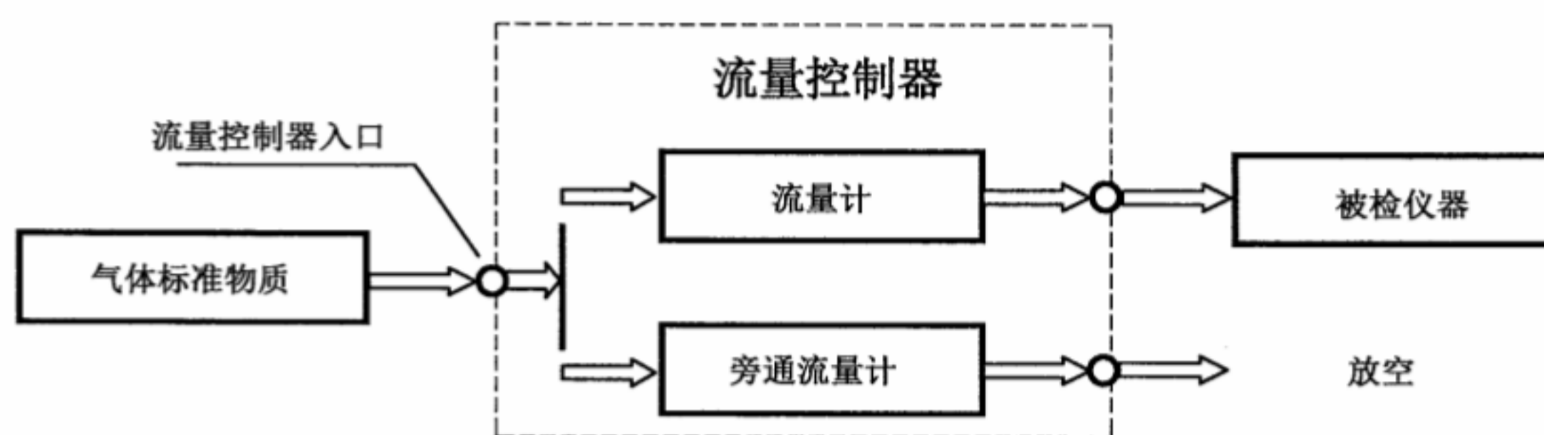
图 1 流量控制器
