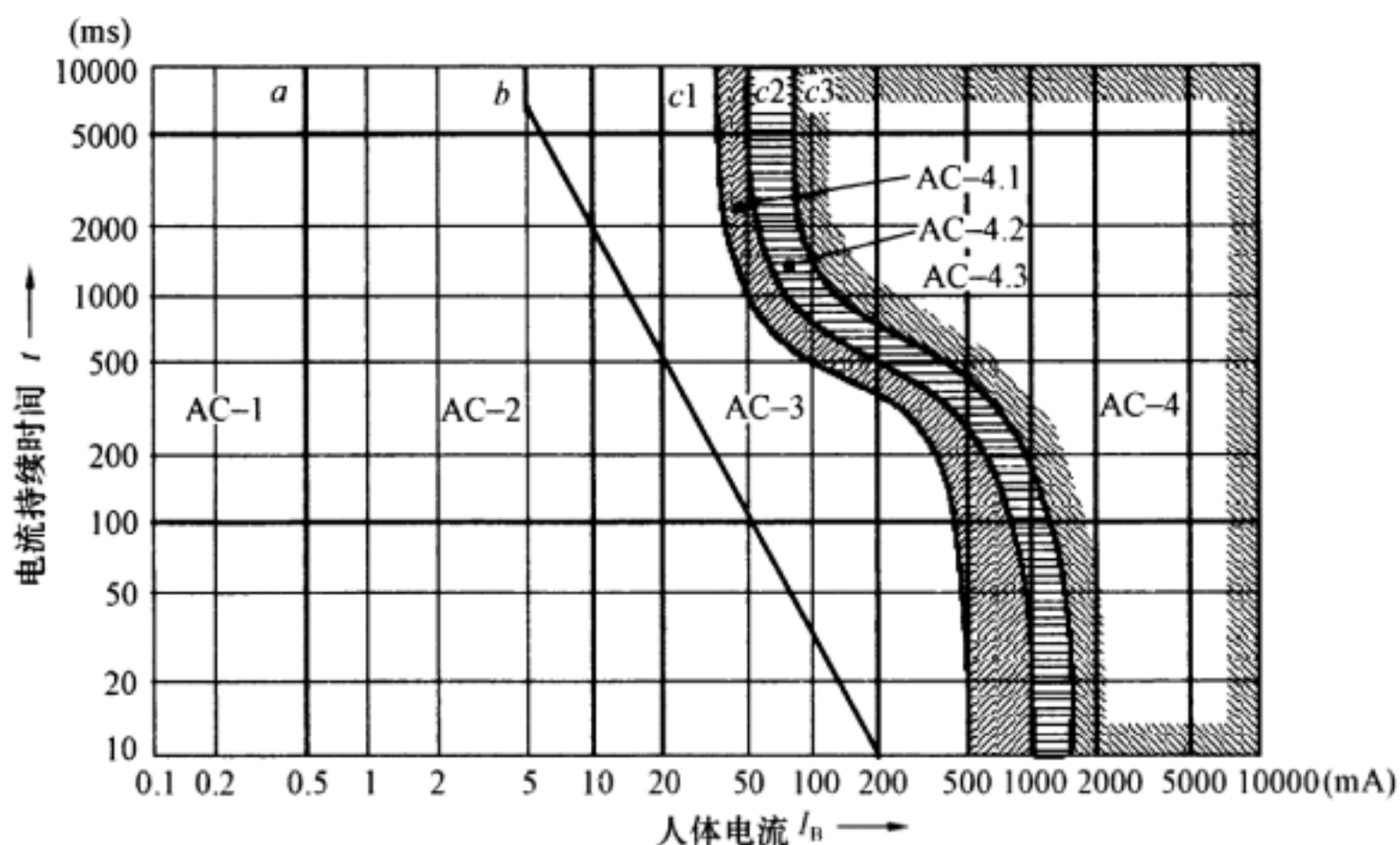
图1 交流电流通过人体时的效应
