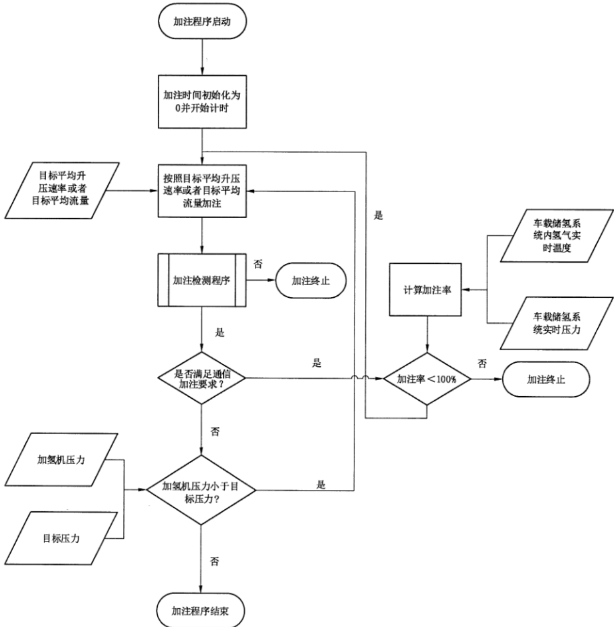
图 B.3 加注程序流程图
