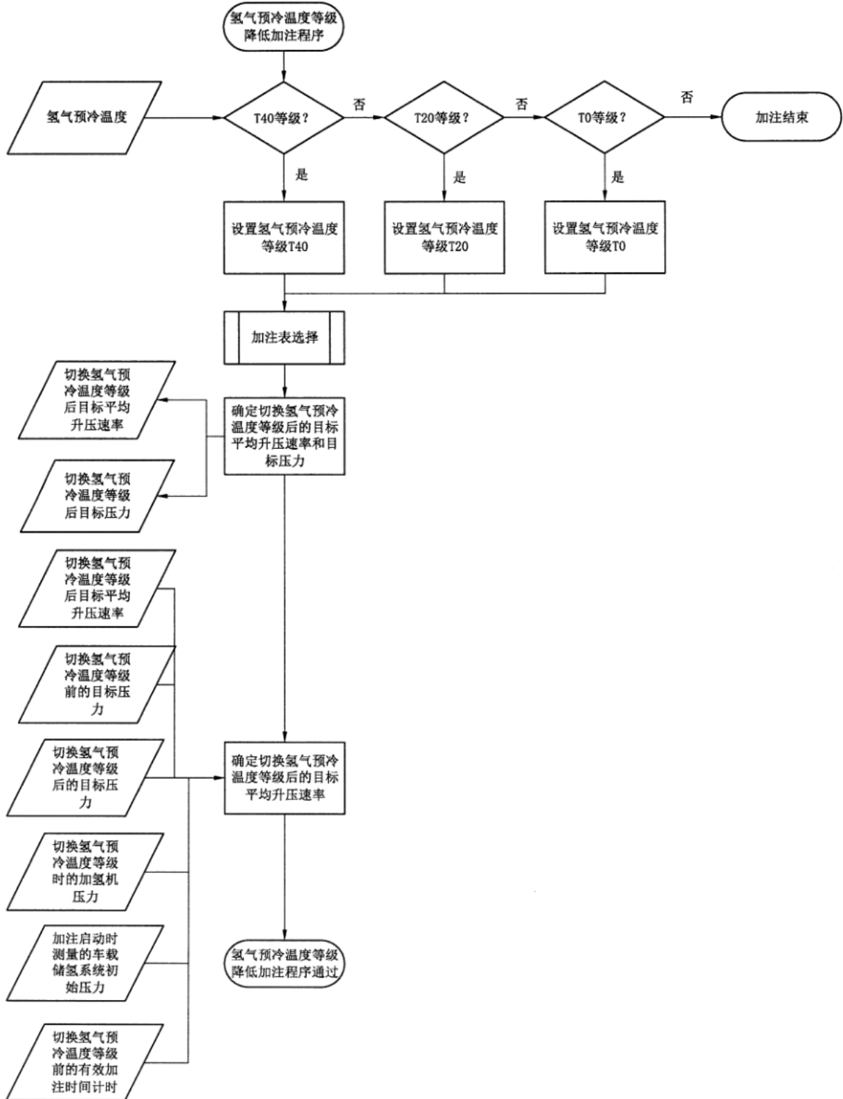
图 B.5 氢气预冷温度等级降低加注程序流程图
