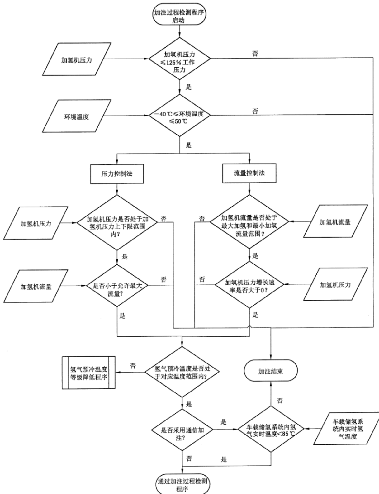
图 B.4 加注过程检测程序流程图
