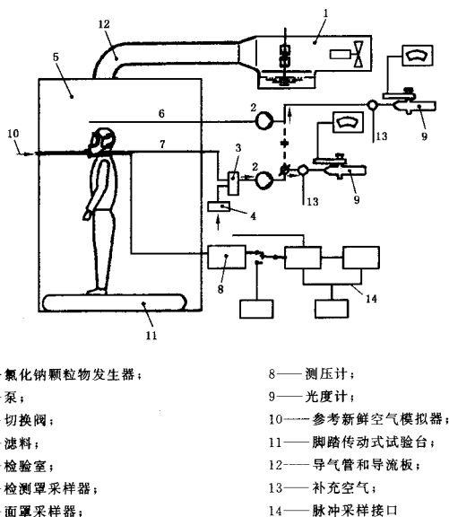
图 E.2 氯化钠定量适合性检验装置示意图
