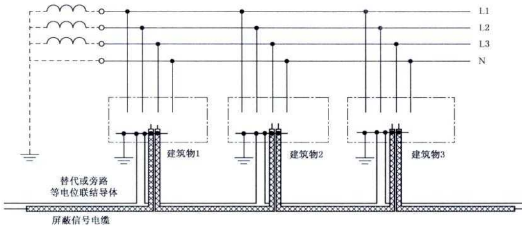
图 44.R2 TT 系统中替代或旁路等电位联结导体的示例
