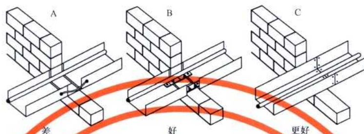
图 44. R22 分断的金属部分连接
