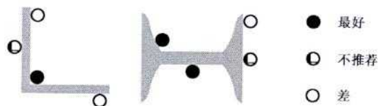
图 44. R21 金属构件内电缆位置
