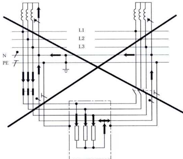
图 44. R9B 在具有不当的三极开关的三相转换供电电源中中性电流流动
