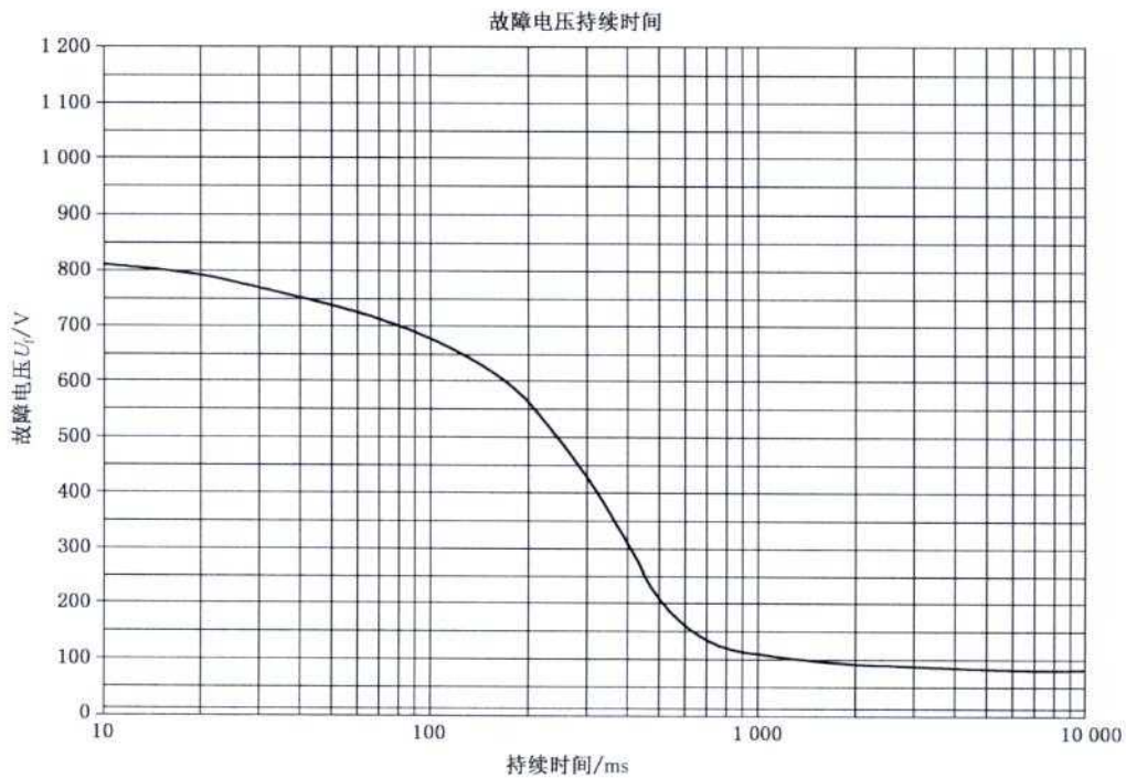
图 44. A2 变电所内高压侧发生接地故障时允许的故障电压值
