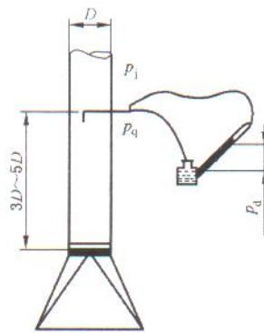
图 A.3 排风罩的排风量和阻力的测定
