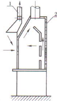
图 12 补风罩
