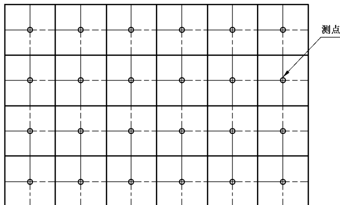
图 5 矩形管道测点位置
