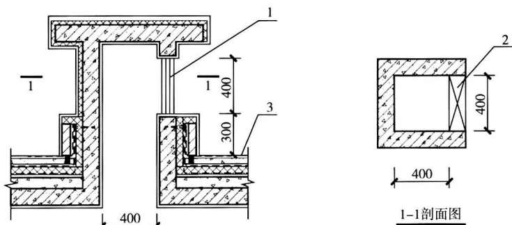
图 4 屋面馈线洞示意图
