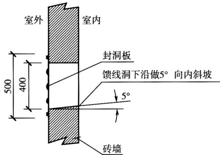
图1 机房孔洞开孔示意图
