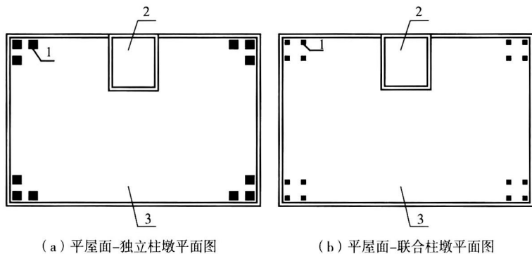
图 6 平屋面支承设施示意图
