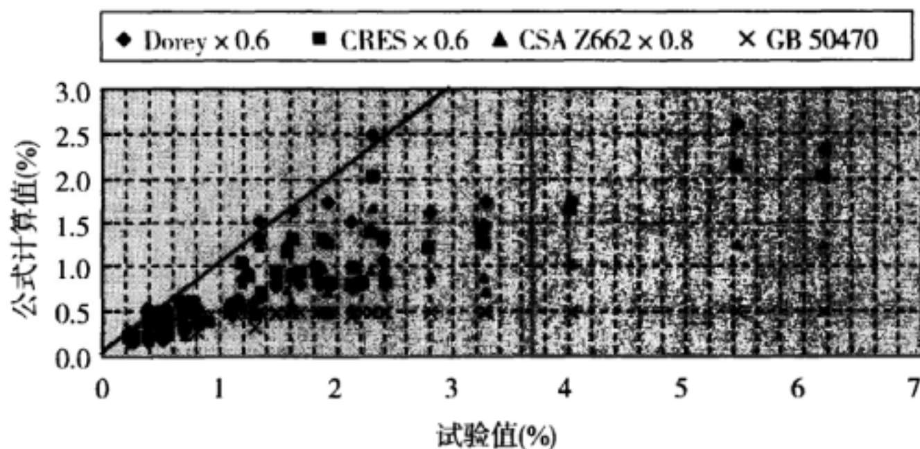
压缩容许应变常用公式对比-所有数据
