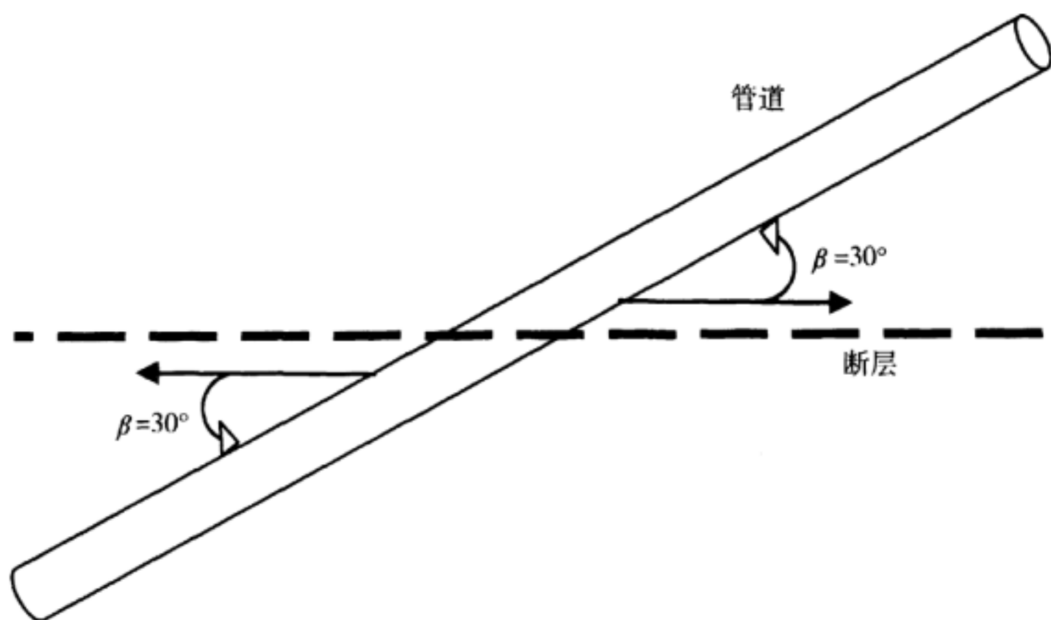
(b) 管道通过右旋走滑断层的交角取值
