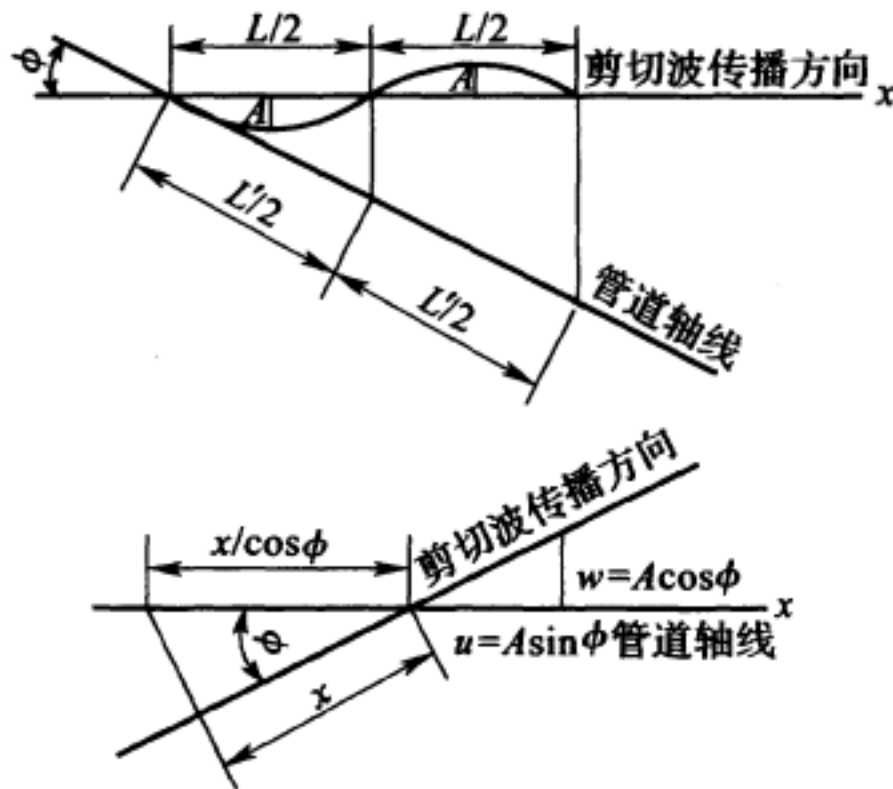
图 4 倾斜的剪切波对管道轴线方向波动的影响
