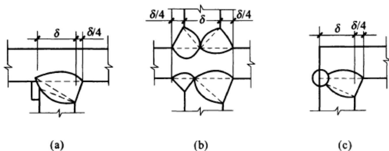
图 8.5.2 焊脚尺寸示意
