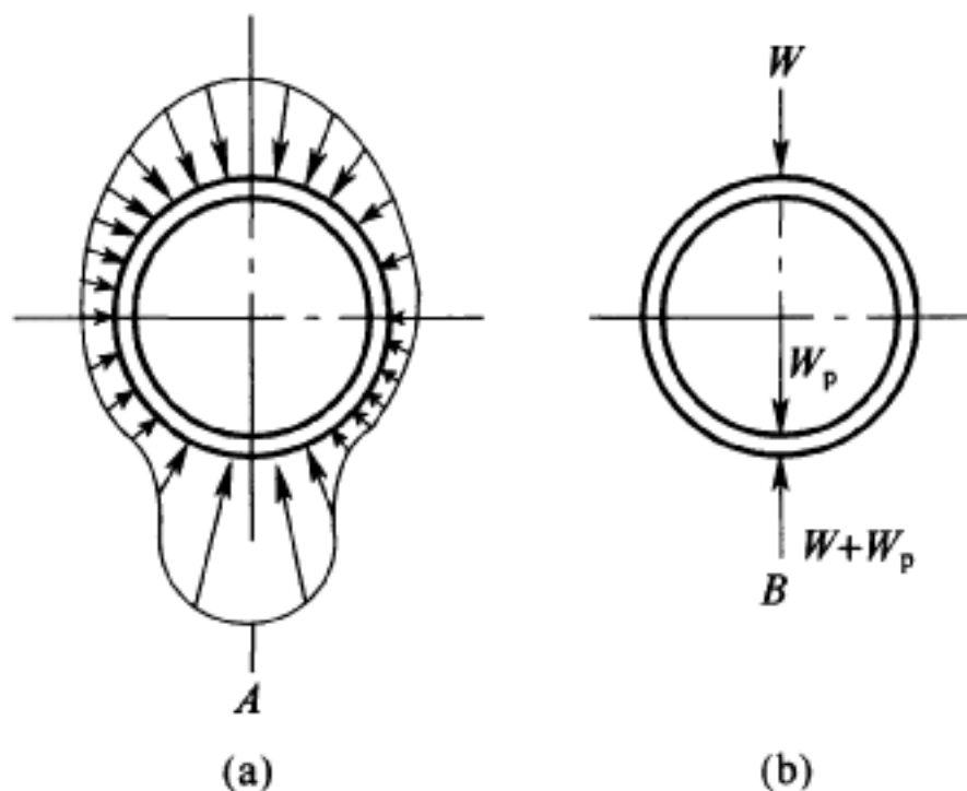
图 7 土压力分布及简化计算图
