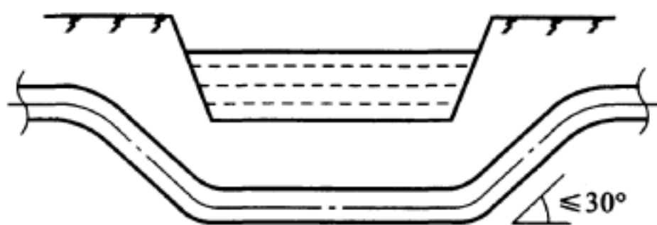
图 7.2.5 直埋式穿越管道示意图
