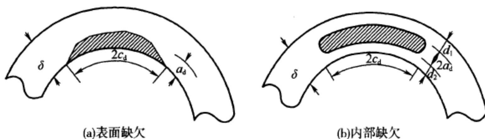
图 D.0.1 环焊缝缺欠类型
