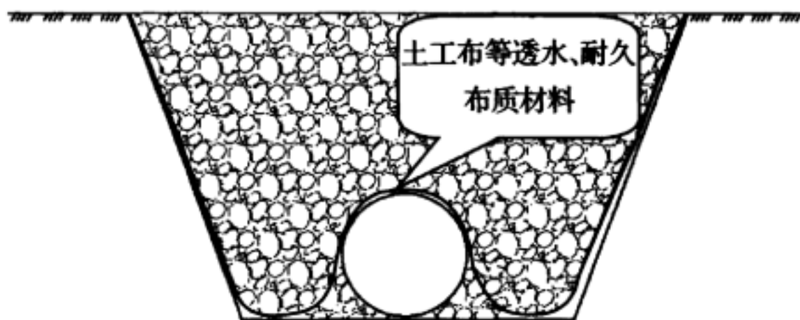
图 12 衬铺压土管沟示意图
