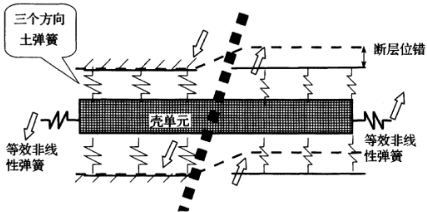
图 11 壳有限元分析模型简图
