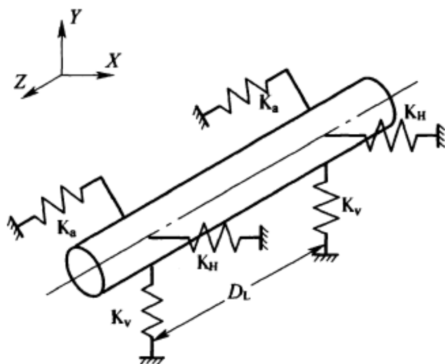
图 E.0.2-1 埋地管道的有限元模型
