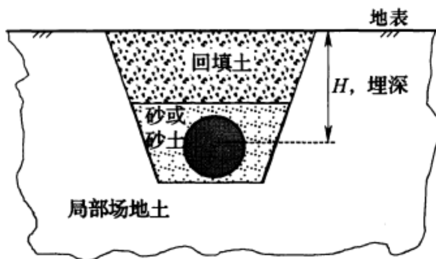
图 10 埋地管道的横向剖面图
