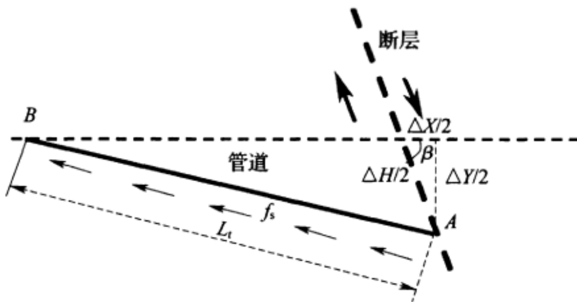
图 8 断层位移对管道的影响
