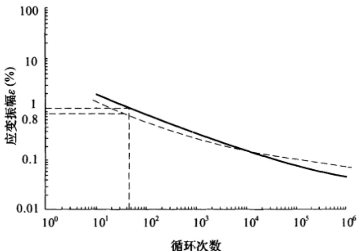
图 3 设计疲劳曲线
