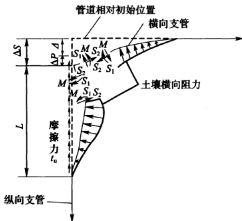
图 5 弯管附近管道受力简图
