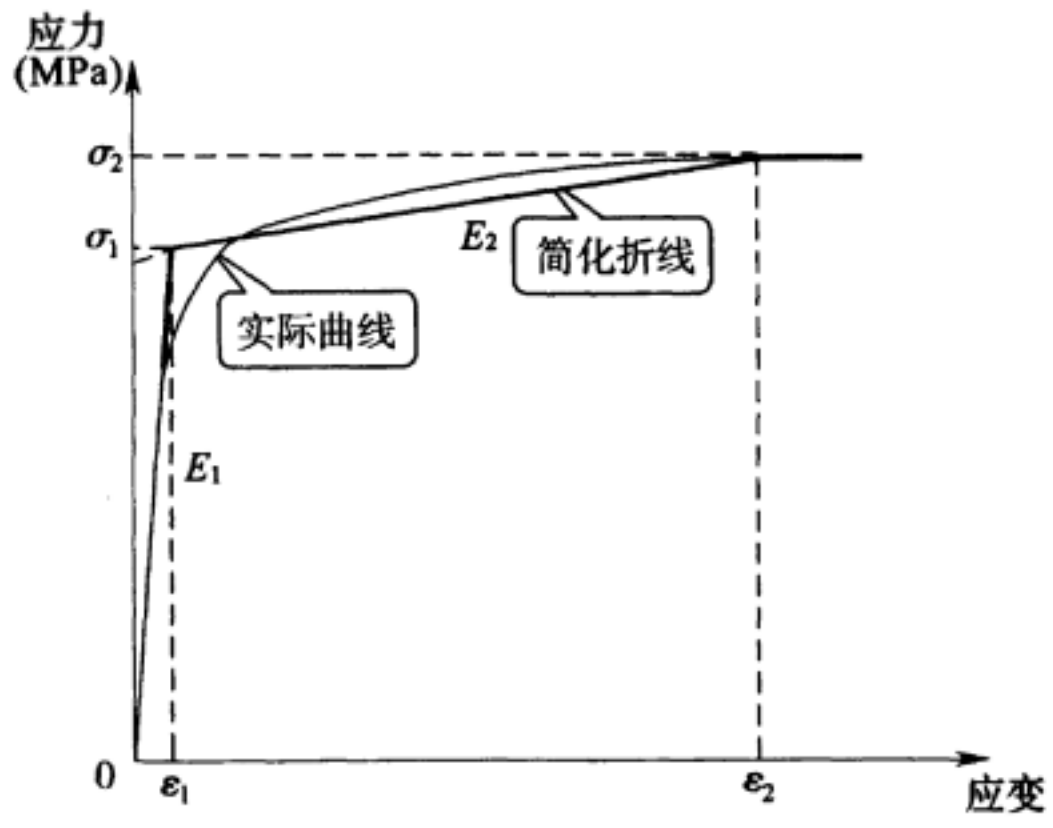
图 C. 0. 4 应力-应变简化折线示意图
