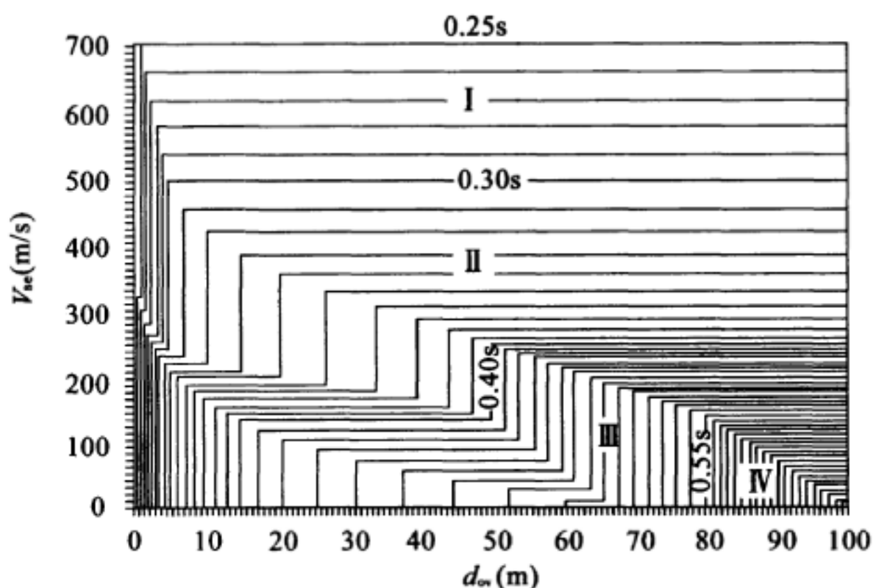
图 2 在 d_{ov} - V_{sc} 平面上的 T_g 等值线图
