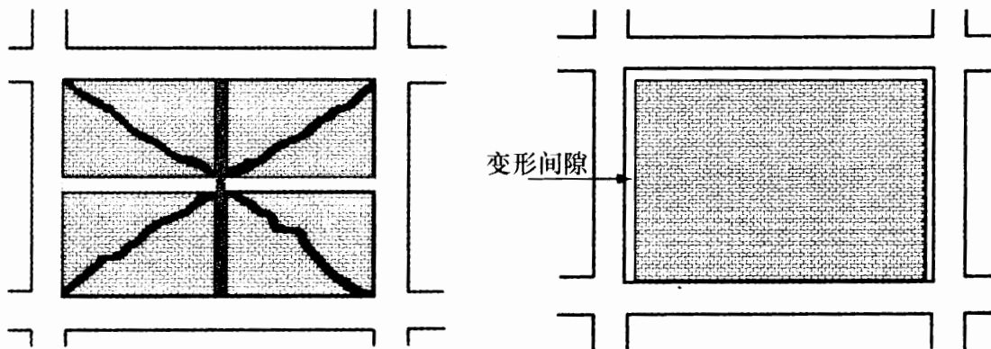
图 1 刚性连接示意图
